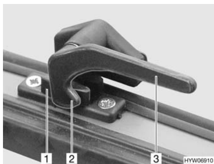
Fig. 33 Leva di serraggio (posizione "Chiusa")
