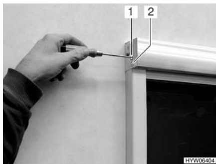
Fig. 139 Regolazione reazione elastica delle molle
