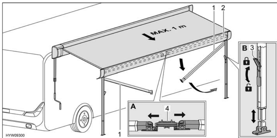
Fig. 25 Preparazione dei montanti di supporto
