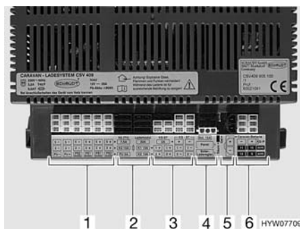
Fig. 81 Apparecchio per l'alimentazione elettrica (CSV 409)
