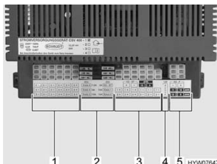
Fig. 79 Apparecchio per l'alimentazione elettrica (CSV 400-1)
