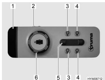
Fig. 13 Telecomando (sistema di manovra)
