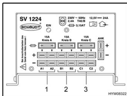
Fig. 80 Apparecchio per l'alimentazione elettrica supplementare (SV 1224)
