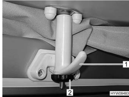
Fig. 46 Tenditore (bloccato)
