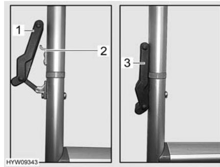
Fig. 48 Cerniera (scaletta di accesso)
