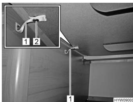
Fig. 56 Fissaggio del piano del tavolo
