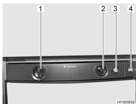
Fig. 114 Elementi di comando (Dometic RMS)
