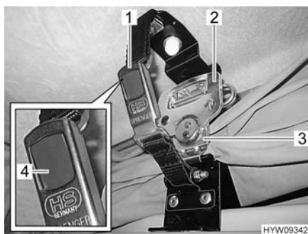
Fig. 54 Bloccaggio (tetto a soffietto)
