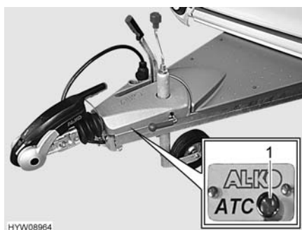
Fig. 5 LED di controllo (sistema per il controllo del rimorchio)
