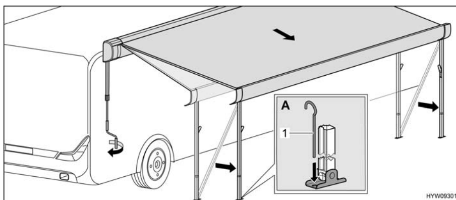
Fig. 26 Collocazione della tenda nella posizione finale
