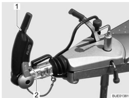
Fig. 129 Indicatore (guarnizioni di attrito davanti e dietro)
