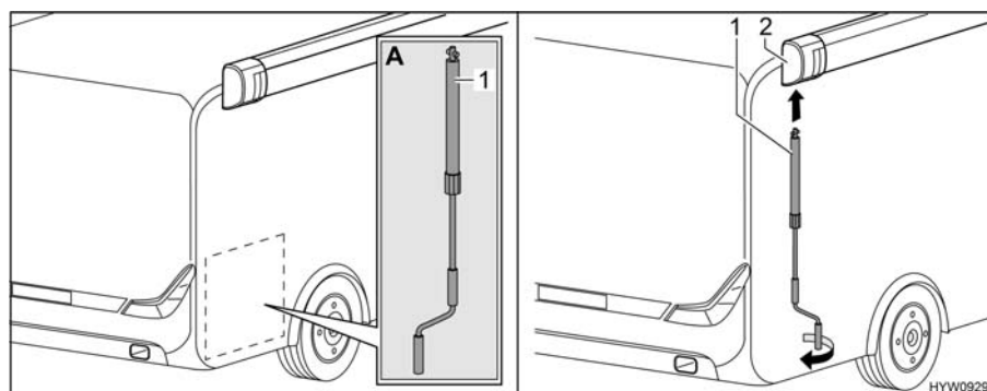
Fig. 24 Applicazione manovella
