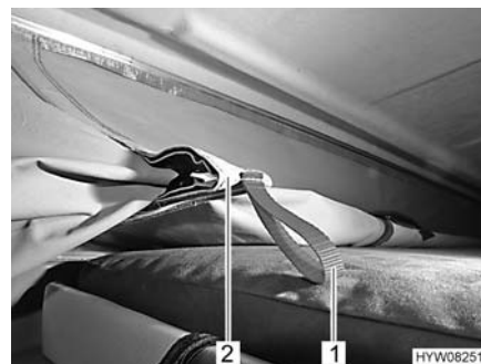
Fig. 53 Dispositivo di inserzione (tetto a soffietto)
