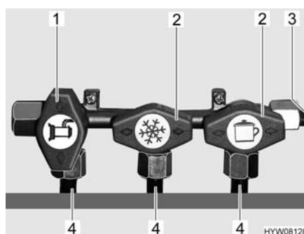
Fig. 75 Posizione dei rubinetti di arresto del gas (esempio)
