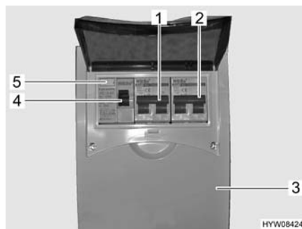
Fig. 90 Scatola dei fusibili a 230 V con interruttore di sicurezza e interruttore automatico FI
