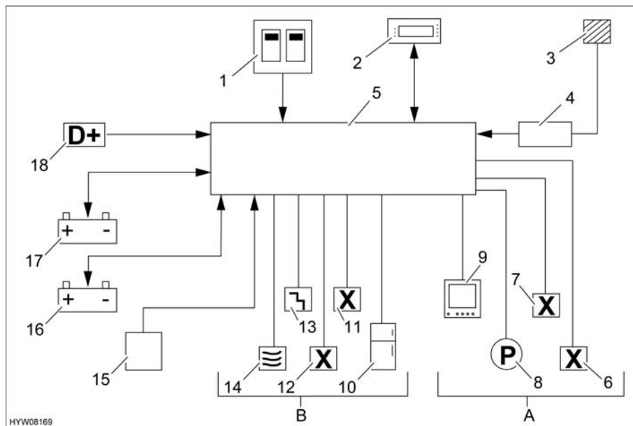
Fig. 92 Schema del cablaggio a 12 V
