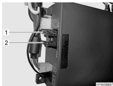
Fig. 89 Apparecchio di controllo impianto TV satellitare
