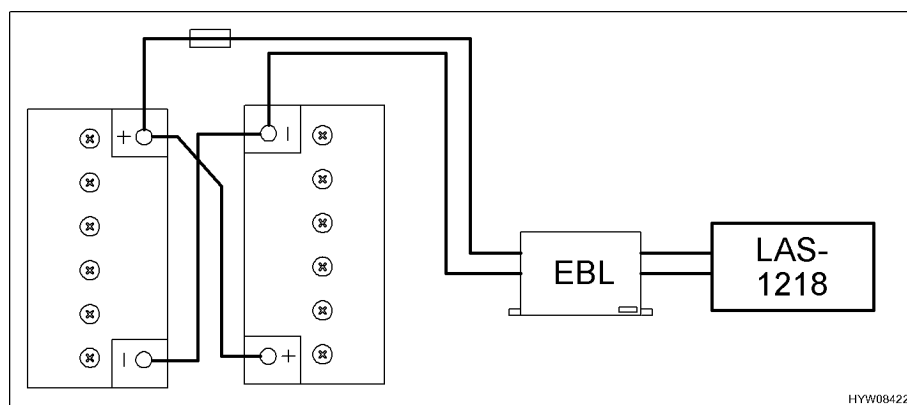
Fig. 81 Collegamento batteria ausiliare
