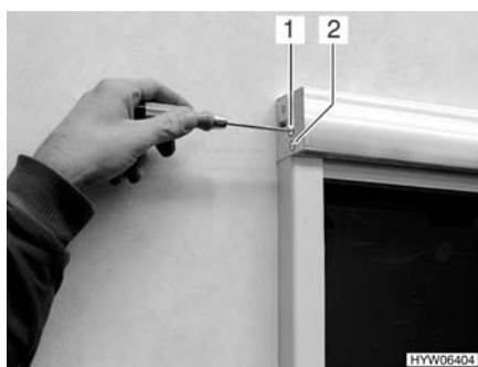
Fig. 123 Regolazione reazione elastica delle molle
