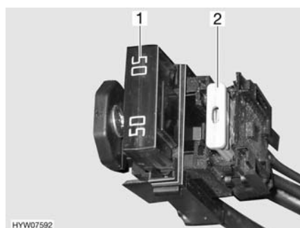
Fig. 86 Fusibili nella batteria di avviamento
