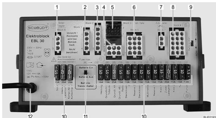
Fig. 82 Centralina elettrica (EBL 30)
