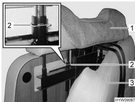
Fig. 59 Rimozione poggiatesta
