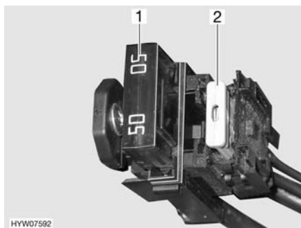
Fig. 87 Fusibili nella batteria dell'abitacolo
