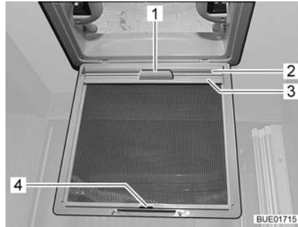
Fig. 41 Oscurante a rullo
