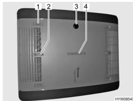
Fig. 102 Indicatore di funzionamento e distribuzione dell'aria
