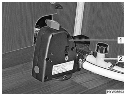
Fig. 122 Rubinetti di scarico e valvola di sicurezza/di scarico
