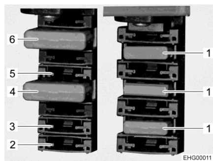
Fig. 98 Fusibili (batteria dell'abitacolo)
