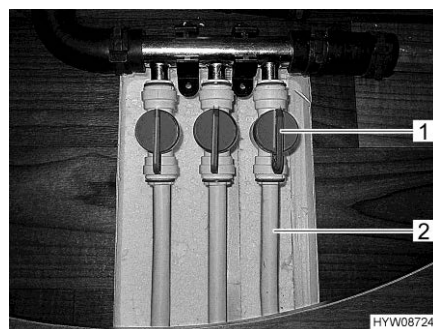
Fig. 127 Valvole di mandata (riscaldamento a pavimento)
