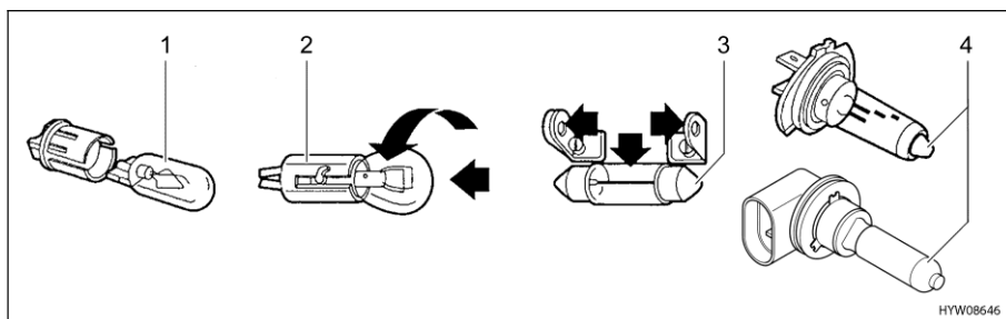
Fig. 180 Tipi di lampade ad incandescenza
