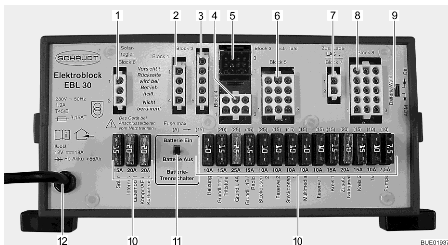
Fig. 91 Centralina elettrica (EBL 30)
