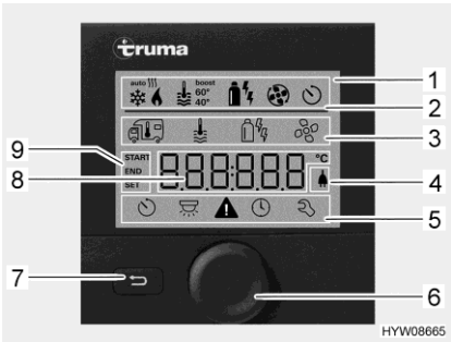
Fig. 111 Centralina di controllo con indicazioni
