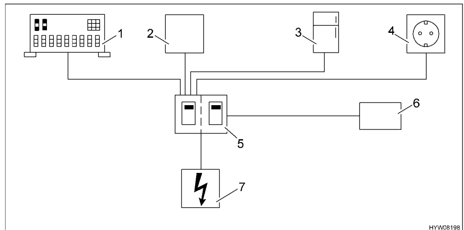
Fig. 106 Schema del cablaggio a 230 V
