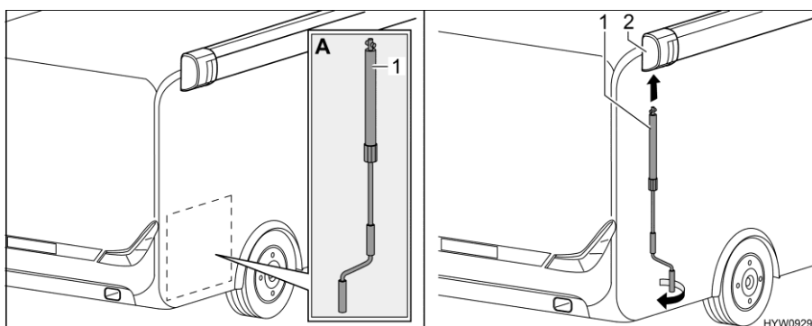
Fig. 27 Applicazione manovella
