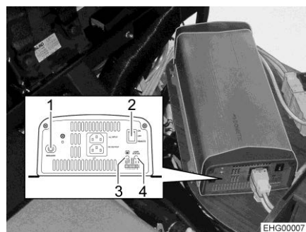
Fig. 92 Invertitore (rappresentazione di esempio)
