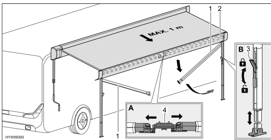
Fig. 28 Preparazione dei montanti di supporto
