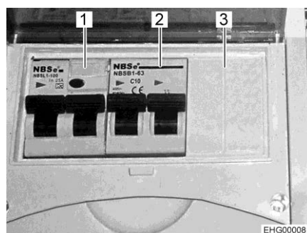
Fig. 93 Scatola dei fusibili supplementare
