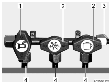
Fig. 76 Posizione dei rubinetti di arresto del gas (esempio)
