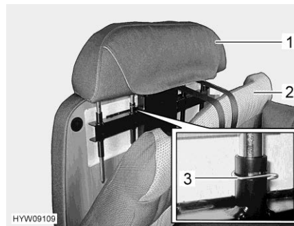
Fig. 20 Regolazione poggiatesta
