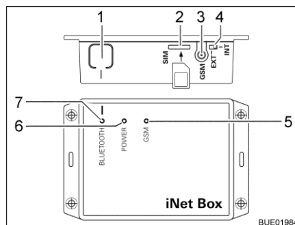
Fig. 114 Truma iNet Box
