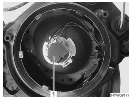
Fig. 215 Lampada ad incandescenza (faro anabbagliante/abbagliante)
