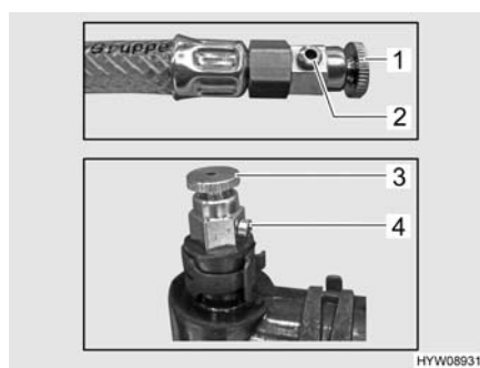
Fig. 209 Valvole di sfiato (riscaldamento ad acqua calda)
