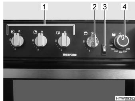
Fig. 175 Elementi di comando (blocco cucina)
