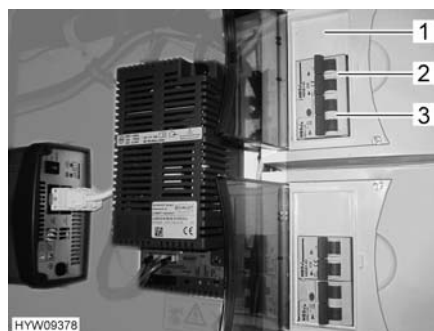
Fig. 126 Scatola dei fusibili supplementare
