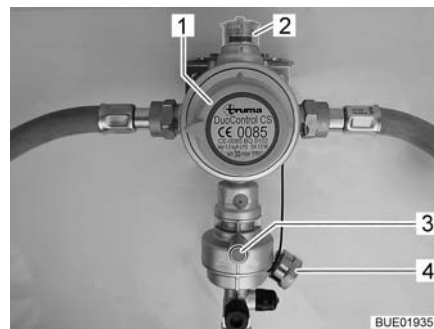
Fig. 117 Impianto di regolazione DuoControl
