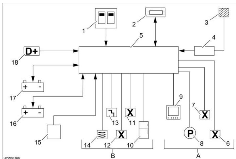
Fig. 141 Schema del cablaggio a 12 V
