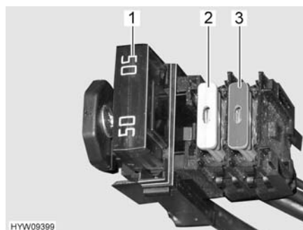
Fig. 131 Fusibili (batteria di avviamento)
