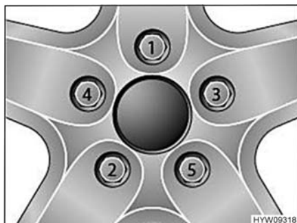
Fig. 224 Serraggio a croce di dadi delle ruote e bulloni delle ruote
