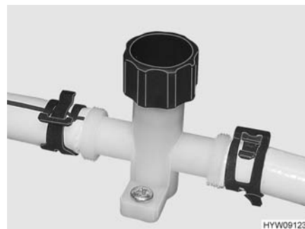
Fig. 203 Rubinetto di scarico (tubatura dell'acqua)
