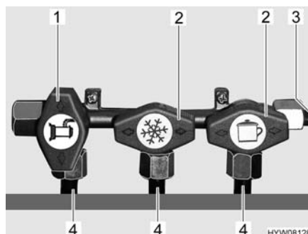
Fig. 111 Posizione dei rubinetti di arresto del gas (esempio)
