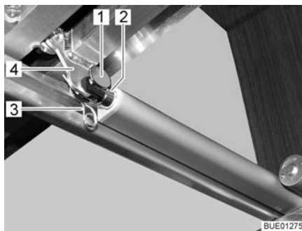
Fig. 101 Azionamento
