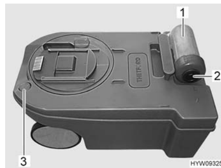
Fig. 201 Serbatoio fecale
