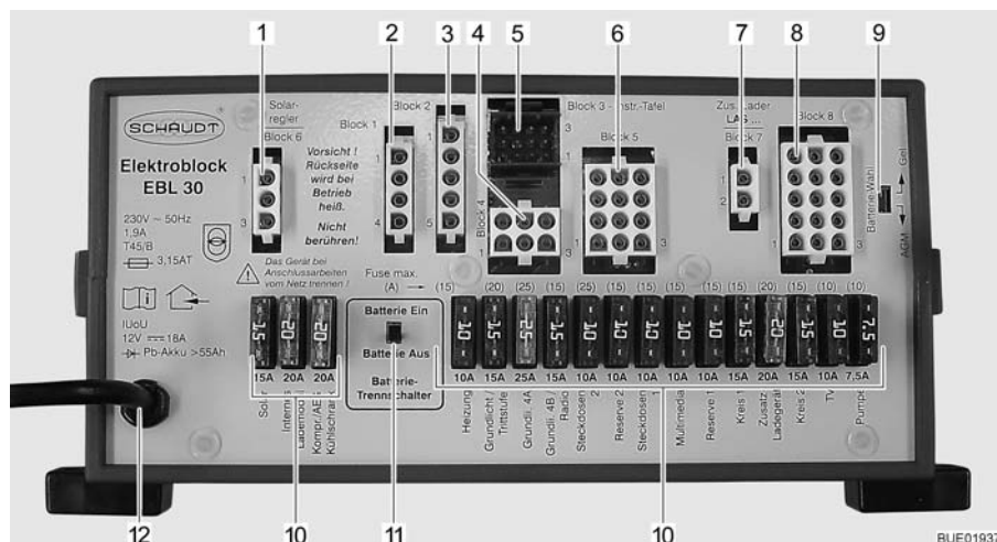
Fig. 124 Centralina elettrica (EBL 30)
