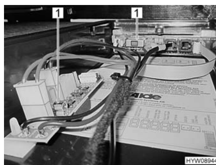
Fig. 134 Fusibili (riscaldamento ad acqua calda)
