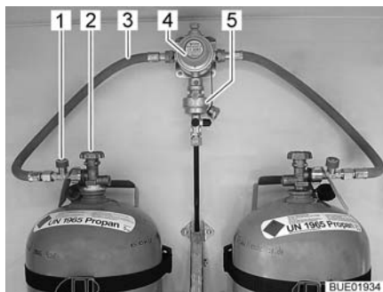
Fig. 116 Bombole del gas con DuoControl
