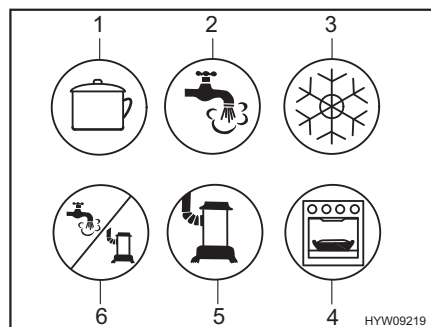
Fig. 142 Simboli dei rubinetti di arresto del gas
