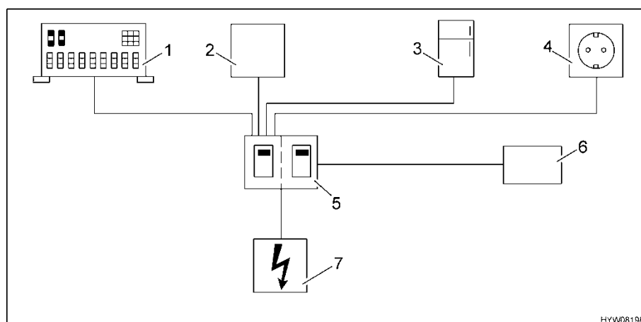
Fig. 140 Schema del cablaggio a 230 V
