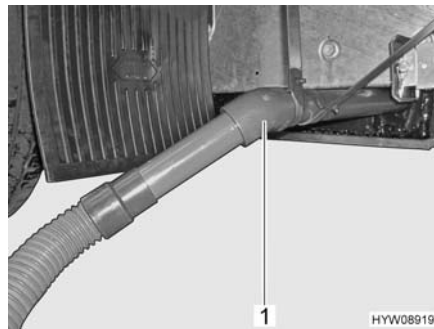
Fig. 193 Tubo di scarico con tubo di gomma per lo scarico
