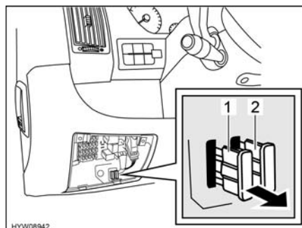
Fig. 133 Fusibili (sospensione pneumatica)
