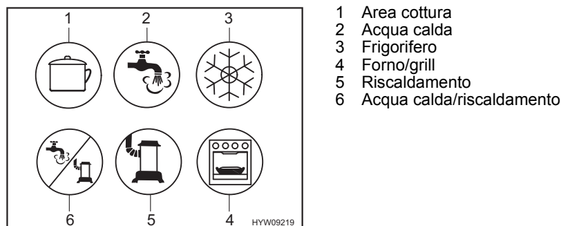
Fig. 110 Possibili simboli dei rubinetti di arresto del gas
