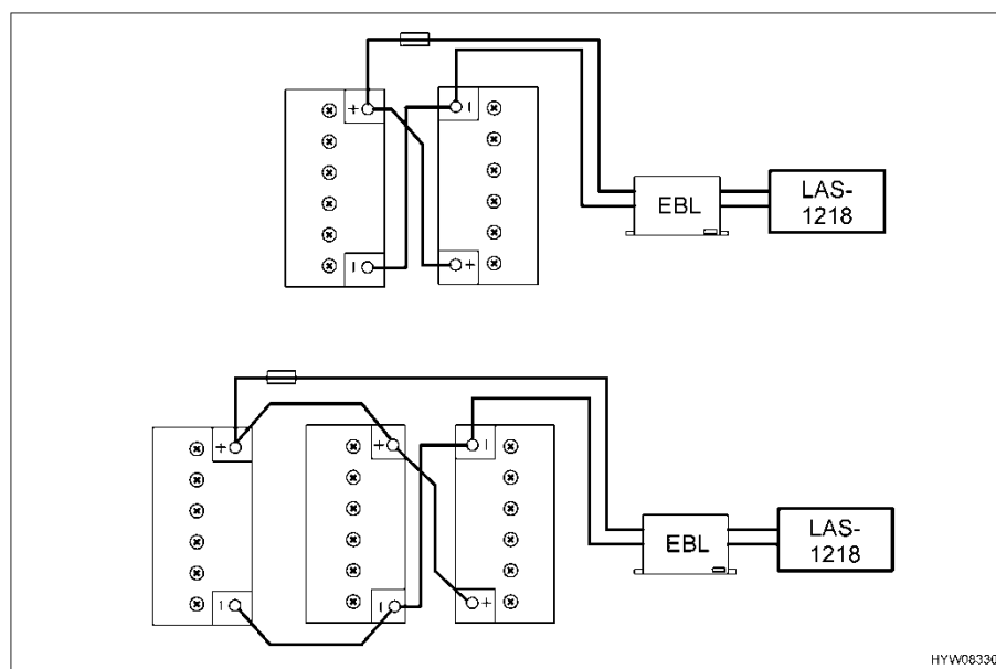
Fig. 123 Collegamento batteria ausiliare
