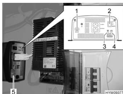
Fig. 125 Invertitore
