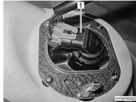
Fig. 217 Luce con regolazione in curva/luce fendinebbia (vista da dietro)
