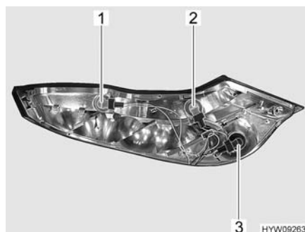
Fig. 219 Unità luci posteriori (smontata)
