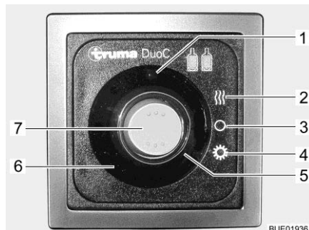
Fig. 117 Centralina di controllo (DuoControl)
