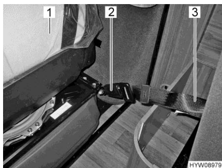
Fig. 29 Fissare il sedile installabile mediante la chiusura della cintura
