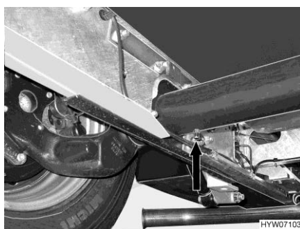
Fig. 228 Asse posteriore AL-KO (Fiat)
