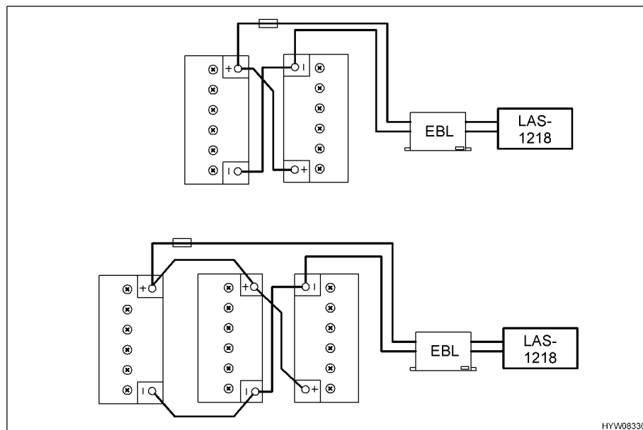
Fig. 121 Collegamento batteria ausiliare
