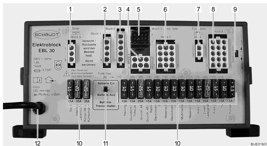
Fig. 122 Centralina elettrica (EBL 30)
