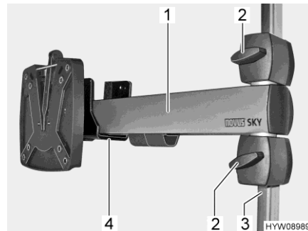
Fig. 89 Supporto dello schermo (raffigurato senza schermo piatto)
