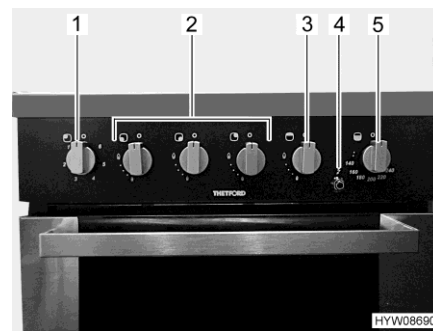
Fig. 168 Elementi di comando (blocco cucina)
