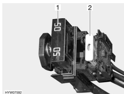
Fig. 126 Fusibili (batteria di avviamento)
