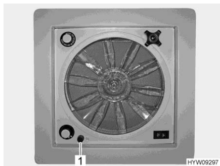
Fig. 132 Fusibile (oblò)
