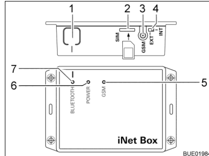
Fig. 162 Truma iNet Box
