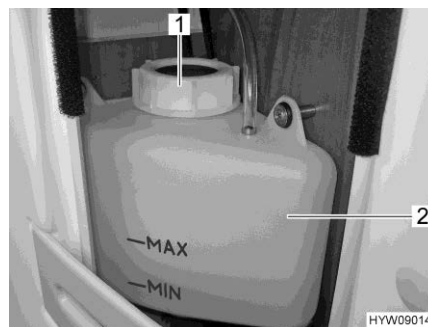
Fig. 213 Vaso d'espansione del riscaldamento ad acqua calda (vano doccia)
