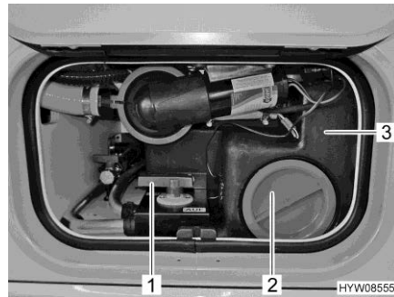
Fig. 202 Serbatoio fecale aggiuntivo
