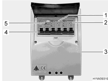
Fig. 124 Interruttore di sicurezza e interruttore automatico FI (scatola dei fusibili a 230 V)
