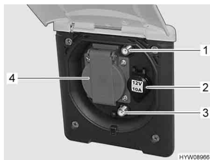
Fig. 80 Presa esterna
