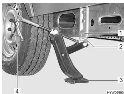
Fig. 137 Cric di AL-KO
