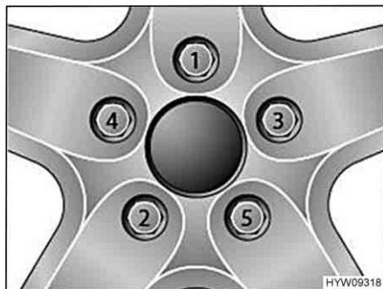
Fig. 133 Serraggio a croce di dadi delle ruote e bulloni delle ruote
