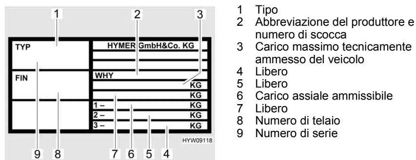
Fig. 131 Targhetta del modello
