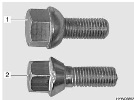
Fig. 134 Bulloni delle ruote
