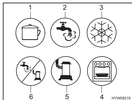
Fig. 87 Simboli dei rubinetti di arresto del gas
