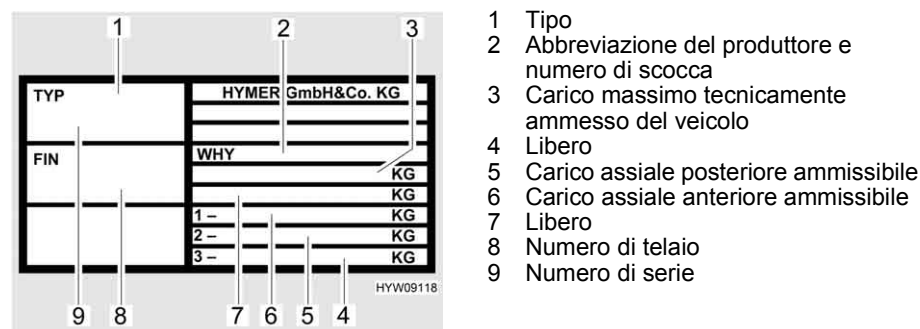
Fig. 140 Targhetta del modello
