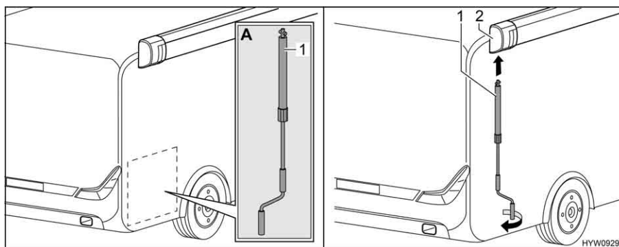
Fig. 27 Applicazione manovella
