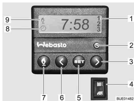
Fig. 136 Centralina di controllo (riscaldamento fisso)
