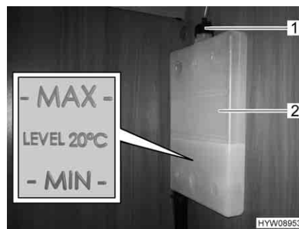
Fig. 189 Riga "MIN/MAX"
