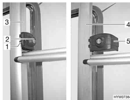
Fig. 2 Bloccaggio (scaletta del portapacchi)
