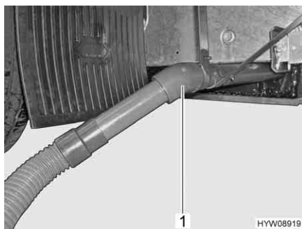
Fig. 171 Tubo di scarico con tubo di gomma per lo scarico
