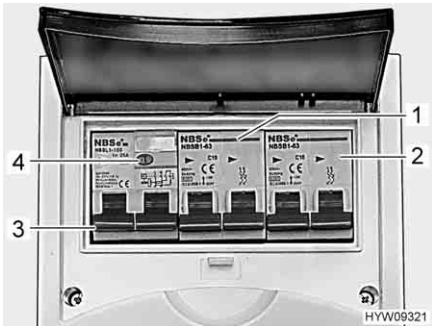
Fig. 110 Interruttore di sicurezza e interruttore automatico FI (scatola dei fusibili a 230 V)
