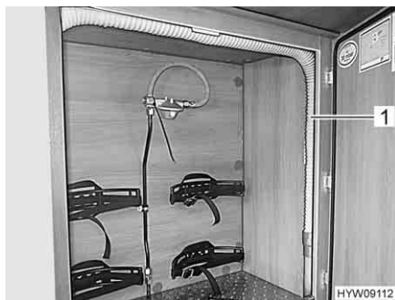
Fig. 169 Tubo di gomma per lo scarico (vano portabombole)
