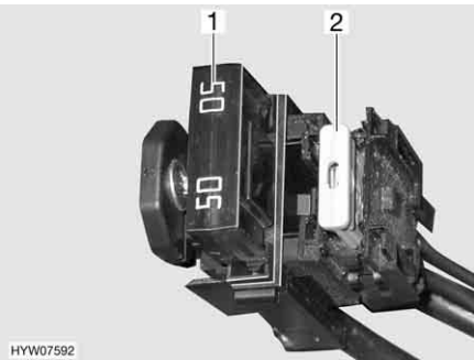
Fig. 105 Fusibili (batteria dell'abitacolo)
