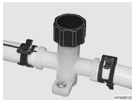
Fig. 184 Rubinetto di scarico (tubatura dell'acqua)
