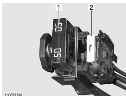
Fig. 104 Fusibili (batteria di avviamento)
