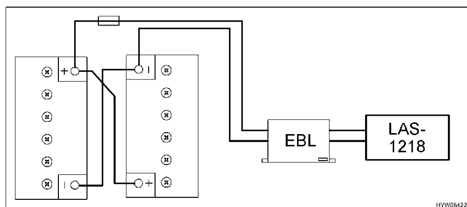
Fig. 99 Collegamento batteria ausiliare
