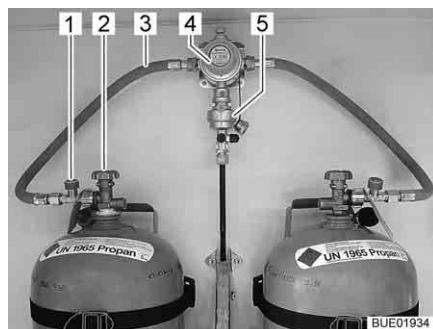
Fig. 92 Bombole del gas con DuoControl
