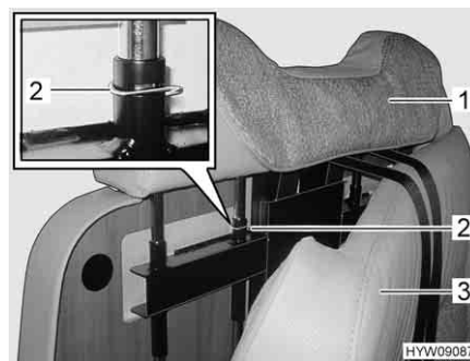
Fig. 67 Rimozione poggiatesta
