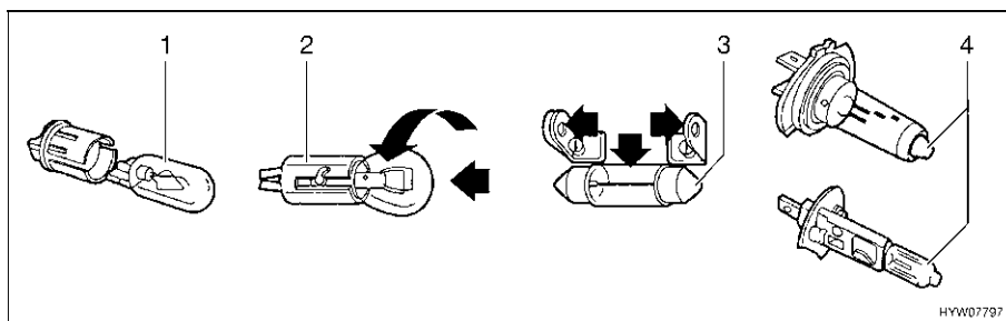
Fig. 191 Tipi di lampade ad incandescenza
