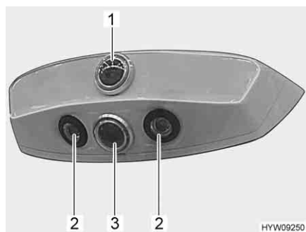
Fig. 21 Modulo telecamere
