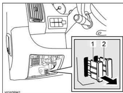
Fig. 97 Fusibili per sospensione pneumatica
