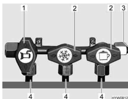
Fig. 79 Posizione dei rubinetti di arresto del gas (esempio)
