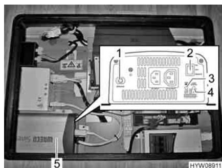
Fig. 88 Invertitore
