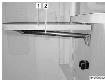
Fig. 66 Tavolo ribaltabile su bancone
