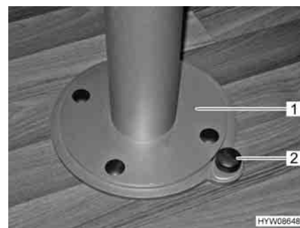
Fig. 63 Sbloccaggio dispositivo di rotazione piede del tavolo
