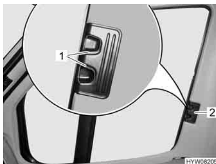
Fig. 49 Tendine oscuranti pieghevoli per il finestrino del conducente/passeggero
