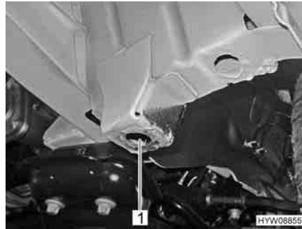
Fig. 193 Punto posizionamento cric (asse anteriore)
