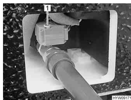
Fig. 165 Azionamento manuale del rubinetto di scolo delle acque grigie
