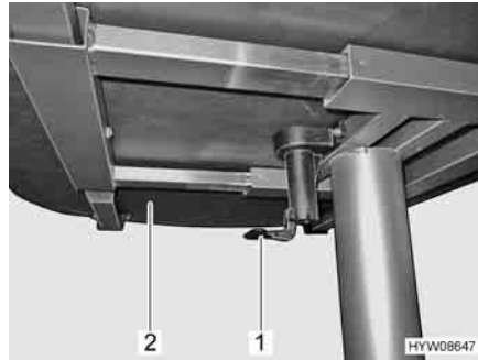
Fig. 64 Leva per spostare il piano del tavolo
