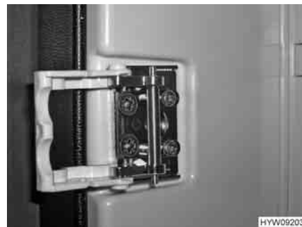
Fig. 151 Dispositivo di chiusura (alternativa) in posizione di ricircolo d'aria
