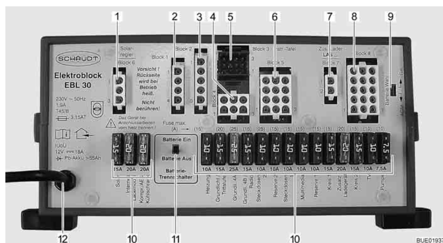
Fig. 87 Centralina elettrica (EBL 30)
