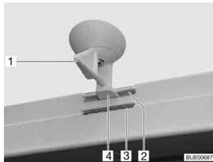
Fig. 50 Oblò inclinabile, bloccaggio
