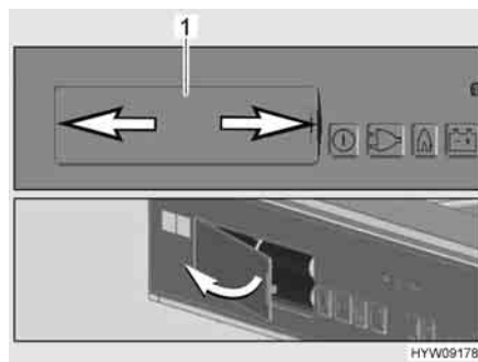
Fig. 143 Vano batteria
