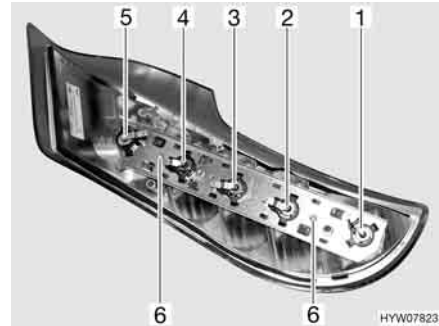
Fig. 185 Luci posteriori (lato posteriore)
