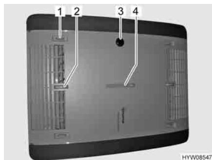
Fig. 123 Indicatore di funzionamento e distribuzione dell'aria
