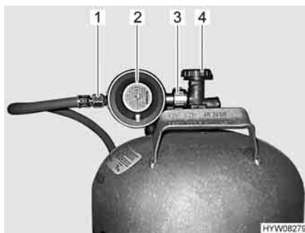
Fig. 84 Raccordo bombola del gas
