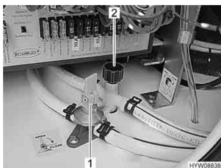
Fig. 126 Rubinetti di scarico
