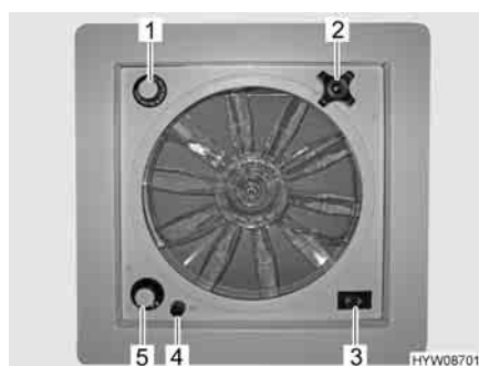
Fig. 56 Oblò con ventilatore
