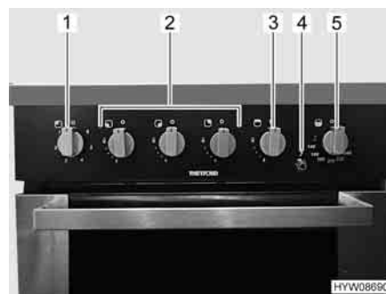
Fig. 134 Elementi di comando del blocco cucina
