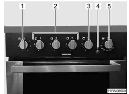
Fig. 173 Elementi di comando del blocco cucina
