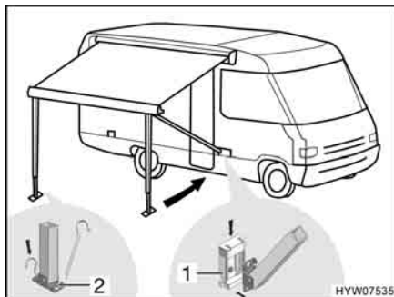
Fig. 53 Fissaggio dei montanti di supporto
