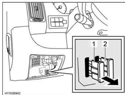
Fig. 133 Fusibili per sospensione pneumatica
