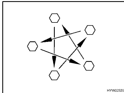
Fig. 237 Serrare a croce i dadi o i bulloni delle ruote
