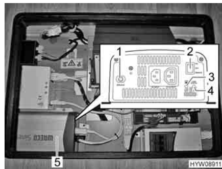
Fig. 124 Invertitore
