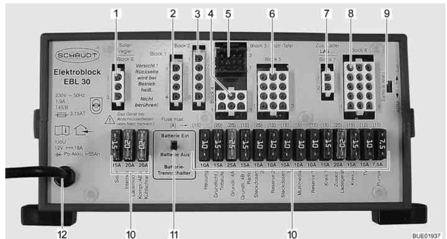
Fig. 123 Centralina elettrica (EBL 30)
