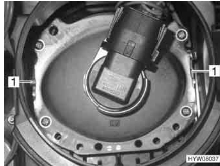
Fig. 226 Conversione fari anteriori
