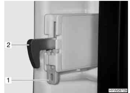
Fig. 184 Fissaggio del gancio di bloccaggio
