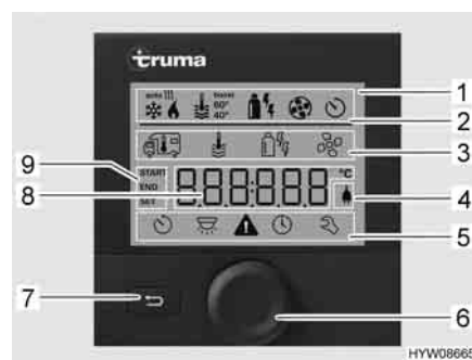
Fig. 142 Centralina di controllo con indicazioni
