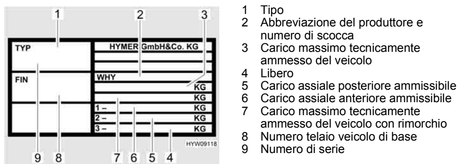
Fig. 234 Targhetta del modello
