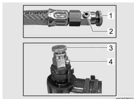
Fig. 219 Valvole di sfiato del riscaldamento ad acqua calda
