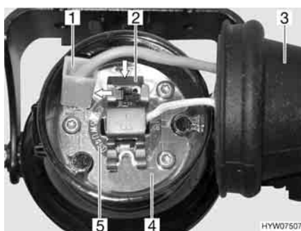
Fig. 225 Luce fendinebbia
