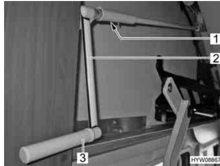
Fig. 75 Manovella per esercizio di emergenza
