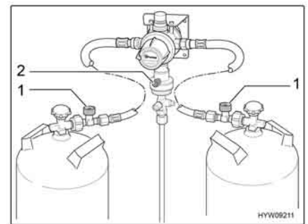
Fig. 16 Regolatore del gas DuoControl
