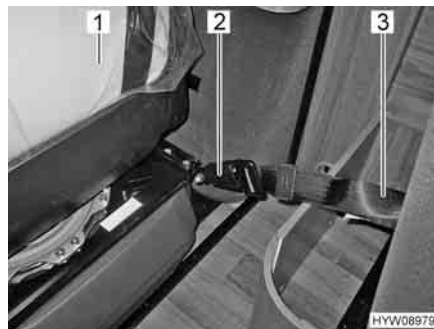
Fig. 35 Fissare il sedile installabile mediante la chiusura della cintura
