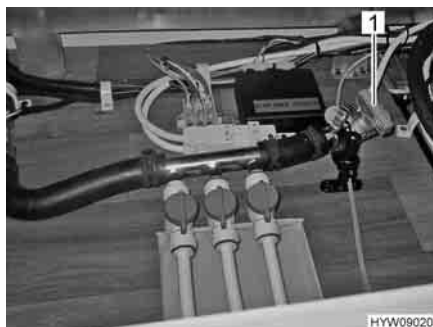
Fig. 216 Attacco per liquido del circuito di riscaldamento
