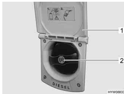
Fig. 47 Bocchettone di riempimento per il rifornimento di carburante
