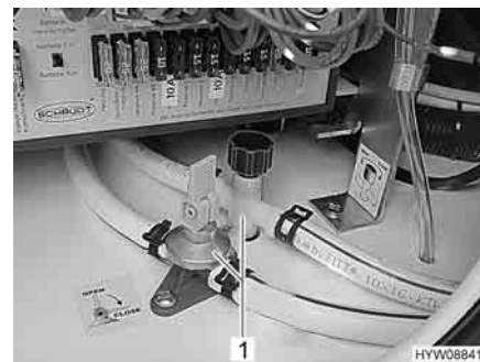
Fig. 195 Rubinetti di scarico (Alde)
