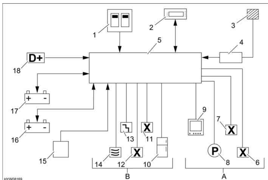
Fig. 138 Schema del cablaggio a 12 V
