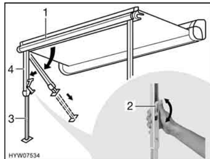
Fig. 52 Installazione dei montanti di supporto
