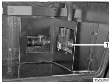
Fig. 148 Scambiatore di calore Alde
