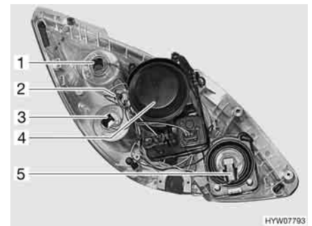
Fig. 224 Fari anteriori (lato posteriore)
