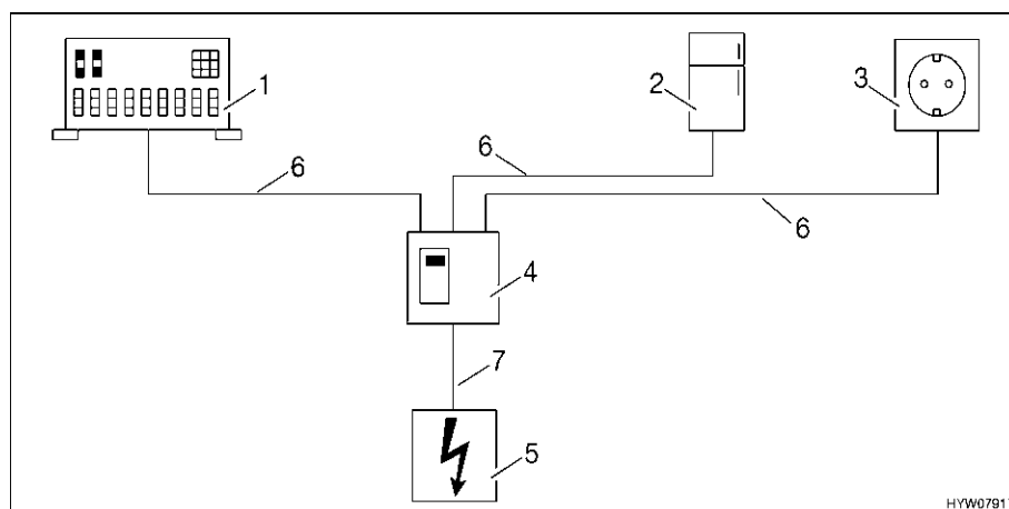
Fig. 51 Schema del cablaggio a 230 V
