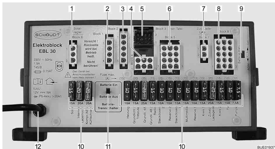
Fig. 43 Centralina elettrica (EBL 30)
