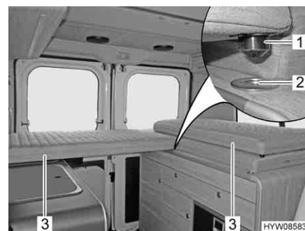
Fig. 33 Fissaggio sul cuscino
