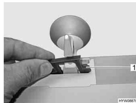
Fig. 55 Sicura contro l'apertura dall'esterno
