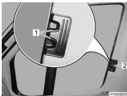
Fig. 50 Tendine oscuranti pieghevoli per il finestrino del conducente/passaggero (Fiat)
