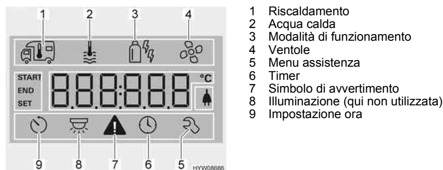
Fig. 126 Display
