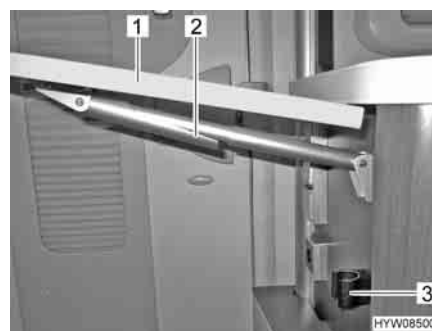
Fig. 69 Chiusura del tavolo ribaltabile su bancone
