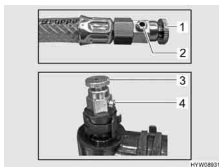
Fig. 184 Valvole di sfiato del riscaldamento ad acqua calda
