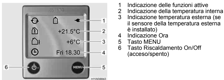
Fig. 111 Centralina di controllo, visualizzazione in stato di inattività
