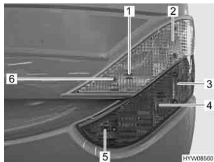
Fig. 190 Luci posteriori (lato anteriore)
