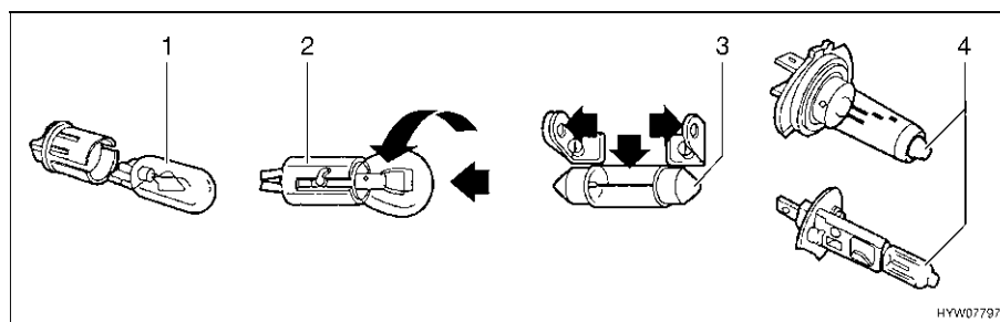
Fig. 185 Tipi di lampade ad incandescenza
