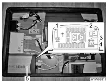
Fig. 90 Invertitore
