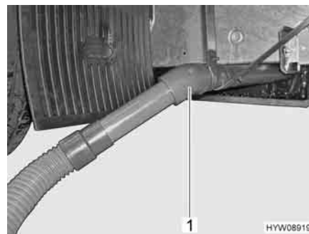
Fig. 164 Tubo di scarico con tubo di gomma per lo scarico
