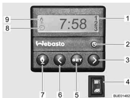
Fig. 121 Centralina di controllo per riscaldamento fisso
