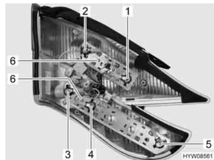
Fig. 191 Luci posteriori (lato posteriore)
