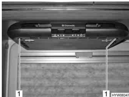
Fig. 180 Svitare la copertura inferiore
