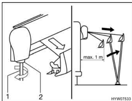
Fig. 29 Estrazione della tenda
