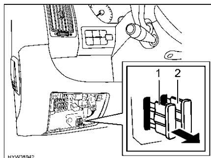
Fig. 99 Fusibili per sospensione pneumatica (Fiat)
