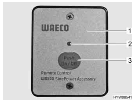
Fig. 92 Interruttore di telecomando
