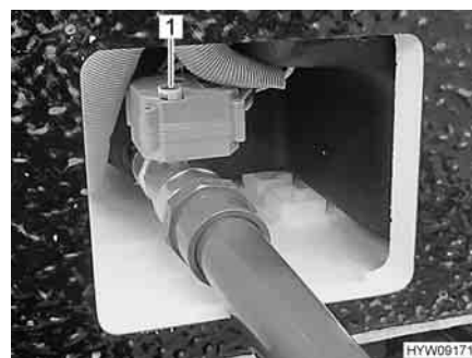
Fig. 168 Azionamento manuale del rubinetto di scolo delle acque grigie
