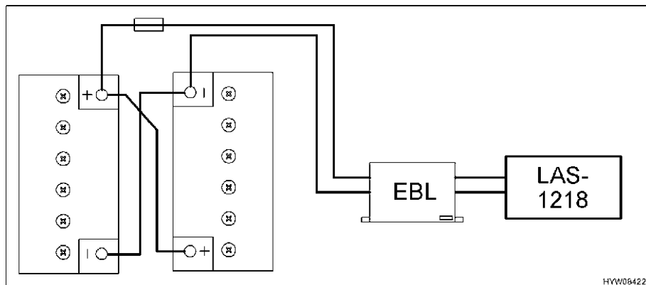
Fig. 88 Collegamento batteria ausiliare
