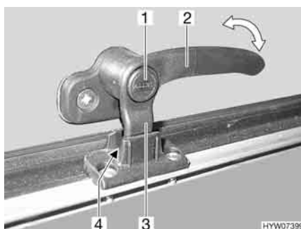
Fig. 41 Leva di serraggio in posizione "Aerazione continua"
