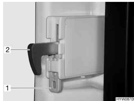
Fig. 102 Fissaggio del gancio di bloccaggio
