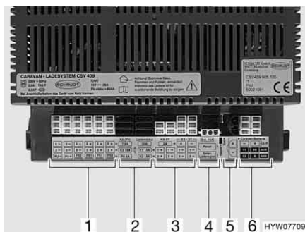
Fig. 67 Apparecchio per l'alimentazione elettrica CSV 409
