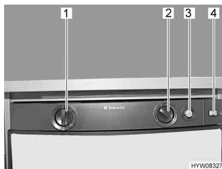
Fig. 100 Elementi di comando per il frigorifero (Dometic RMS)
