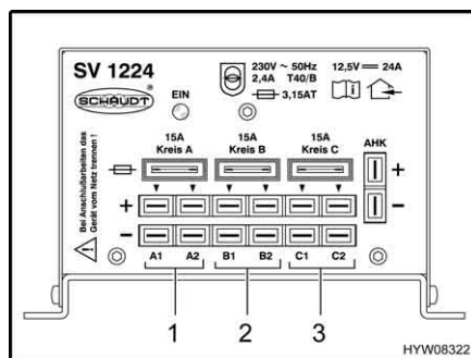
Fig. 66 Apparecchio per l'alimentazione elettrica supplementare SV 1224
