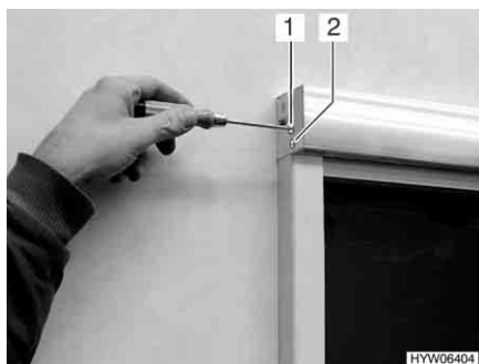
Fig. 127 Regolazione reazione elastica delle molle
