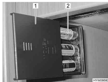
Fig. 126 Sostituzione della batteria
