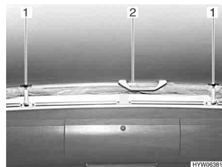
Fig. 36 Tetto sollevabile, chiuso
