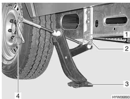
Fig. 134 Cric di AL-KO
