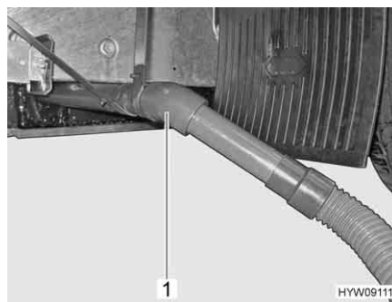
Fig. 92 Tubo di scarico con tubo di gomma per lo scarico
