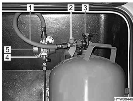
Fig. 50 Raccordo bombola del gas
