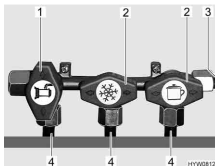
Fig. 52 Posizione dei rubinetti di arresto del gas (esempio)
