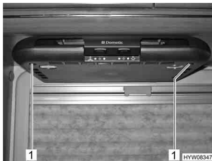
Fig. 102 Svitare la copertura inferiore
