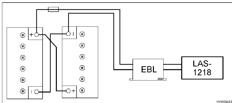
Fig. 58 Collegamento batteria ausiliare
