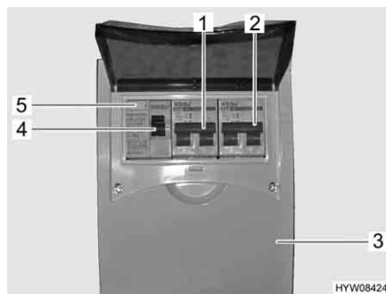
Fig. 66 Scatola dei fusibili a 230 V con interruttore di sicurezza e inter- ruttore automatico FI
