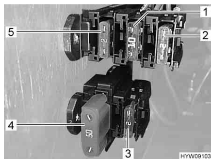
Fig. 64 Portafusibile nella batteria dell'abitacolo
