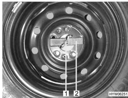
Fig. 170 Ruota di scorta nel gavone di coda
