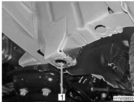
Fig. 168 Punto posizionamento cric (asse anteriore)
