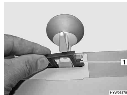
Fig. 43 Sicura contro l'apertura dall'esterno
