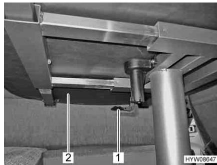
Fig. 54 Leva per spostare il piano del tavolo
