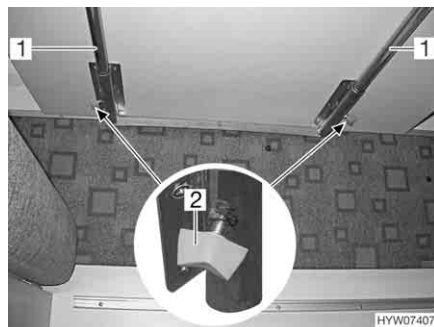
Fig. 57 Tavolo sospeso, bloccaggio della base estraibile
