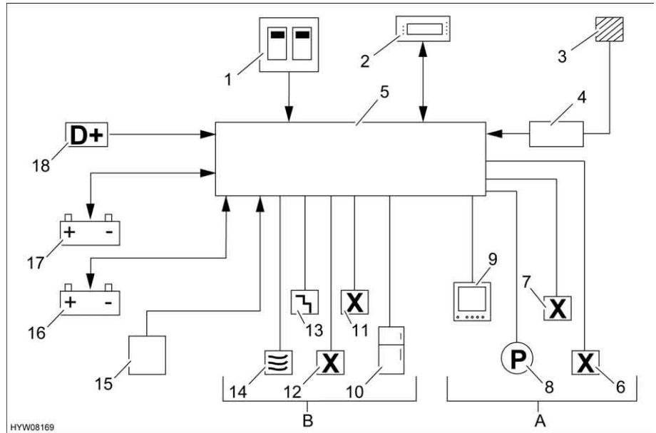
Fig. 97 Schema del cablaggio a 12 V
