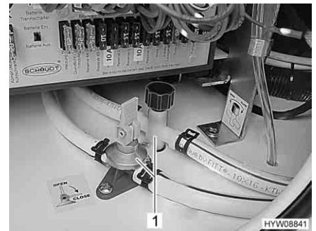
Fig. 151 Rubinetti di scarico (Alde)
