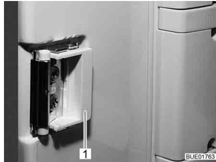
Fig. 132 Dispositivo di chiusura in posizione normale
