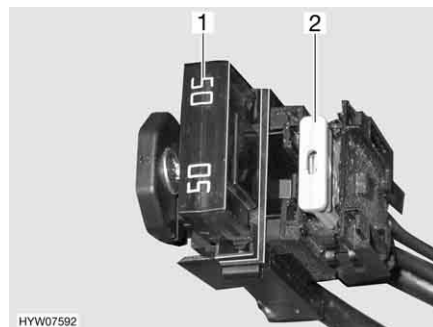
Fig. 91 Fusibili nella batteria di avviamento
