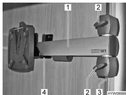
Fig. 9 Braccio snodato per schermo piatto
