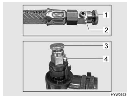
Fig. 154 Valvole di sfiato del riscaldamento ad acqua calda
