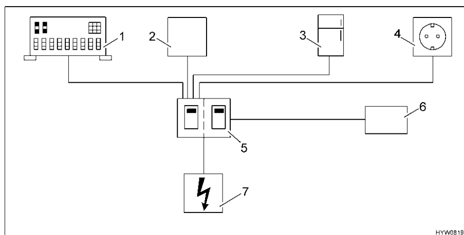
Fig. 96 Schema del cablaggio a 230 V
