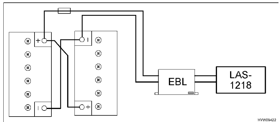
Fig. 86 Collegamento batteria ausiliare
