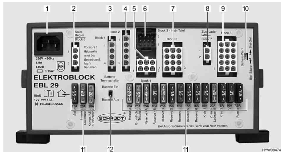
Fig. 87 Centralina elettrica (EBL 29)
