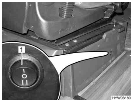
Fig. 110 Interruttore per ventola aggiuntiva
