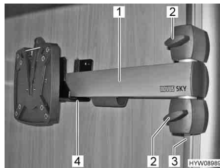
Fig. 59 Supporto dello schermo (raffigurato senza schermo piatto)
