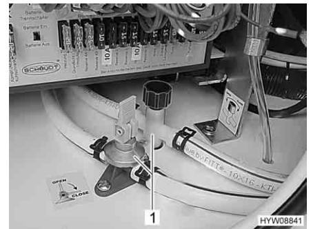
Fig. 138 Rubinetti di scarico (Alde)
