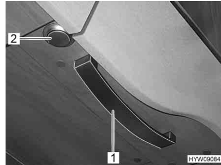
Fig. 13 Bloccaggio del vano abbassabile
