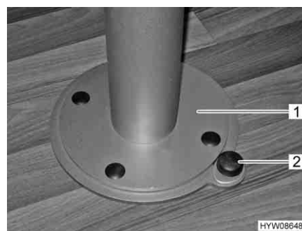
Fig. 58 Sbloccaggio dispositivo di rotazione piede del tavolo
