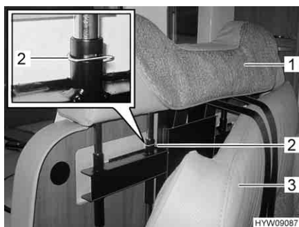
Fig. 68 Rimozione poggiatesta
