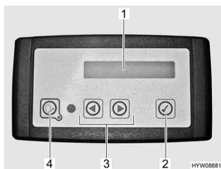
Fig. 64 Frontalino dell'impianto satellitare
