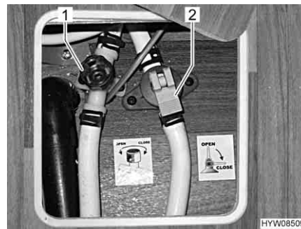
Fig. 127 Rubinetti di scarico (alternativa)
