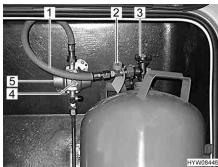
Fig. 83 Raccordo bombola del gas
