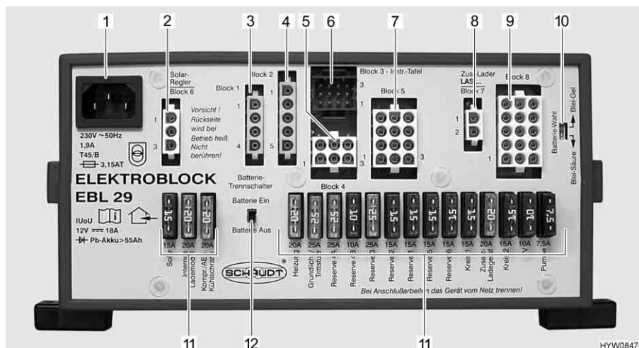
Fig. 92 Centralina elettrica (EBL 29)
