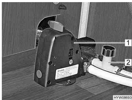
Fig. 160 Rubinetti di scarico e valvola di sicurezza/di scarico
