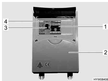
Fig. 94 Scatola dei fusibili a 230 V con interruttore di sicurezza e interruttore automatico FI
