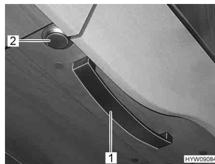
Fig. 14 Bloccaggio del vano abbassabile
