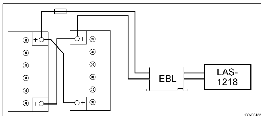
Fig. 91 Collegamento batteria ausiliare
