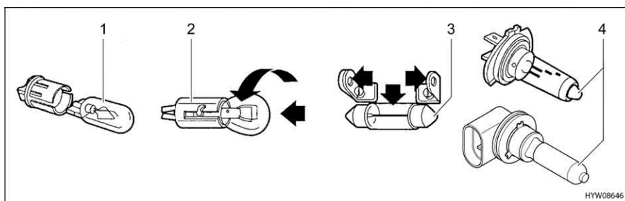
Fig. 186 Tipi di lampade ad incandescenza
