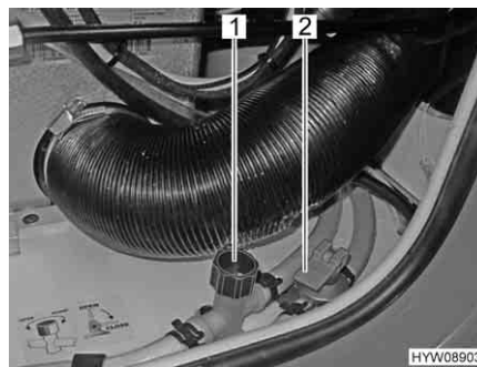
Fig. 147 Rubinetti di scarico
