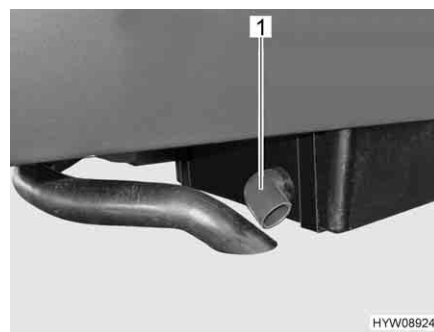
Fig. 174 Tubo di scarico del serbatoio fecale aggiuntivo
