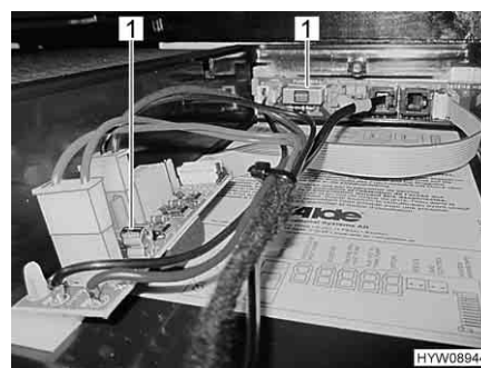
Fig. 126 Fusibili
