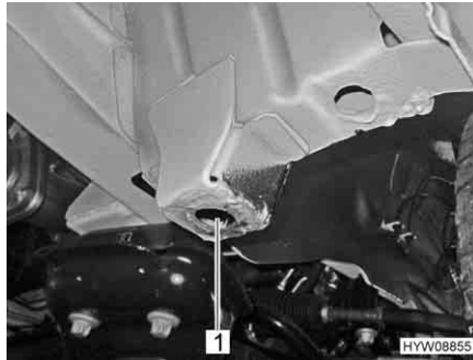
Fig. 205 Punto posizionamento cric (asse anteriore)
