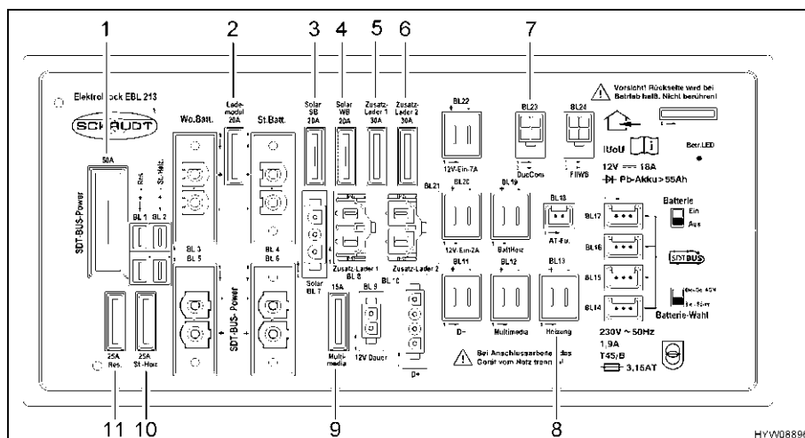
Fig. 123 Fusibili su EBL 213
