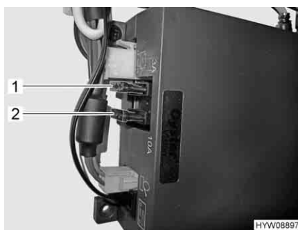
Fig. 127 Apparecchio di controllo impianto TV satellitare
