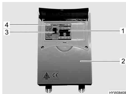
Fig. 118 Scatola dei fusibili a 230 V con interruttore di sicurezza e interruttore automatico FI
