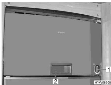
Fig. 152 Forno a gas integrato al frigorifero
