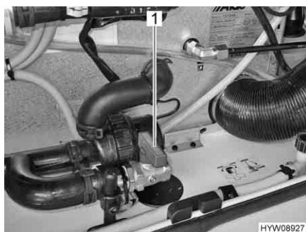
Fig. 180 Attacco per liquido del circuito di riscaldamento
