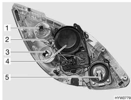
Fig. 189 Fari anteriori (lato posteriore)
