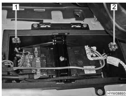
Fig. 120 Fusibili nella batteria di avviamento
