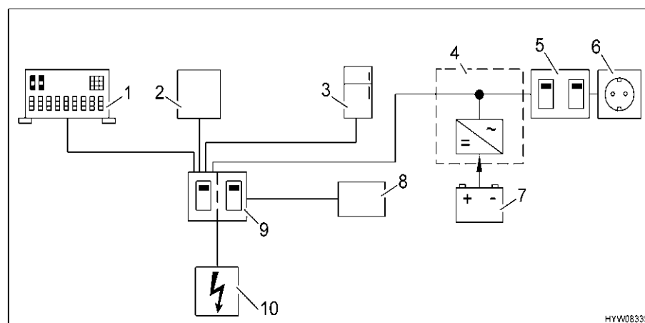
Fig. 130 Schema del cablaggio a 230 V (con invertitore)
