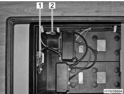
Fig. 121 Fusibili nella batteria dell'abitacolo
