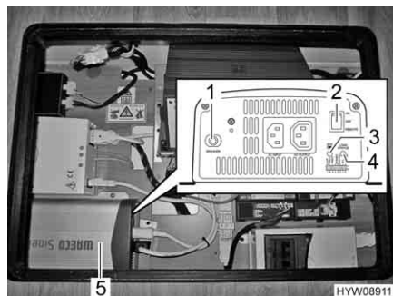
Fig. 113 Invertitore
