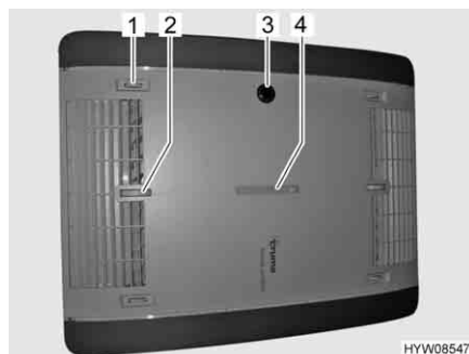
Fig. 144 Indicatore di funzionamento e distribuzione dell'aria
