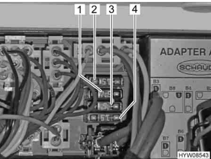
Fig. 122 Box relè AD03
