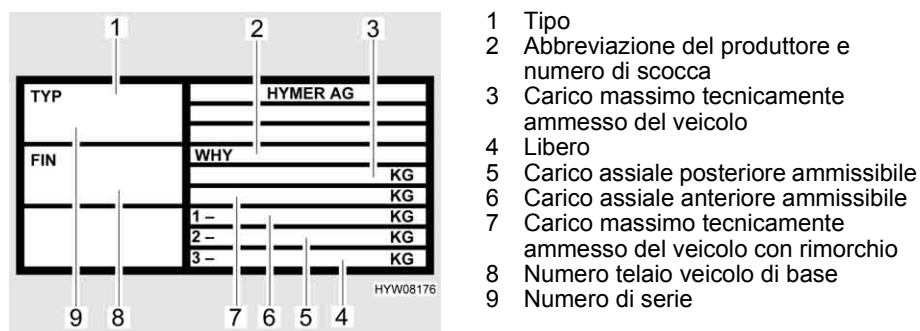
Fig. 200 Targhetta del modello
