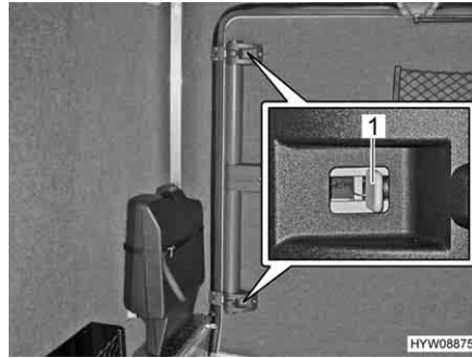
Fig. 43 Porta del garage, sbloccaggio di emergenza dall'interno
