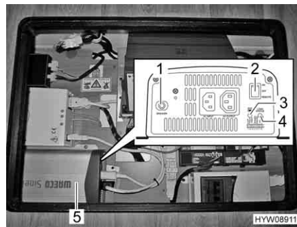
Fig. 101 Invertitore
