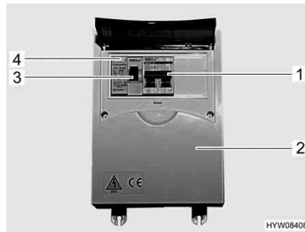
Fig. 105 Scatola dei fusibili a 230 V con interruttore di sicurezza e interruttore automatico FI
