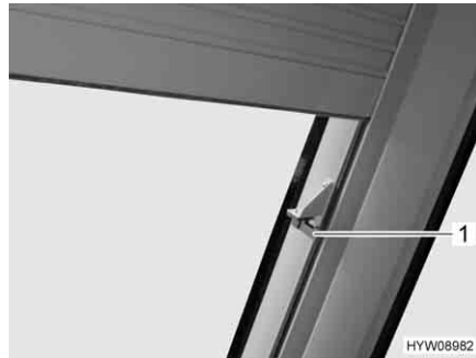
Fig. 28 Chiusure di sicurezza aggiuntive per oscurante a rullo
