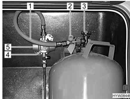
Fig. 91 Vano portabombole
