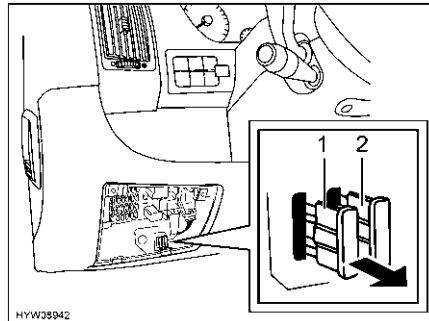
Fig. 110 Fusibili per sospensione pneumatica
