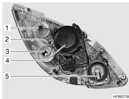
Fig. 165 Fari anteriori (lato posteriore)
