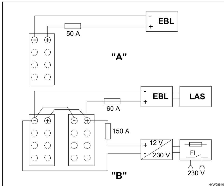
Fig. 99 Collegamento batteria dell'abitacolo
