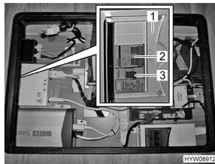
Fig. 102 Scatola dei fusibili supplementare
