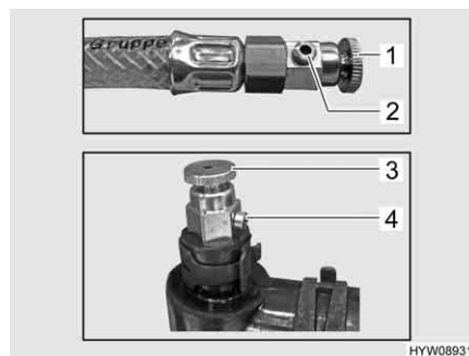
Fig. 160 Valvole di sfiato del riscaldamento ad acqua calda
