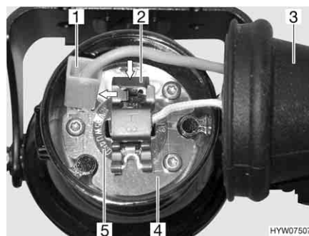
Fig. 166 Luce fendinebbia
