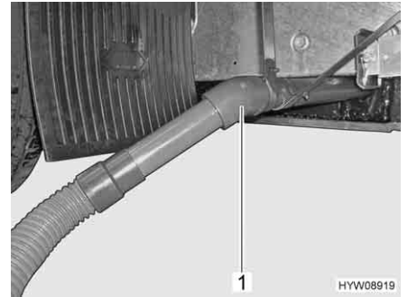
Fig. 149 Tubo di scarico con tubo di gomma per lo scarico
