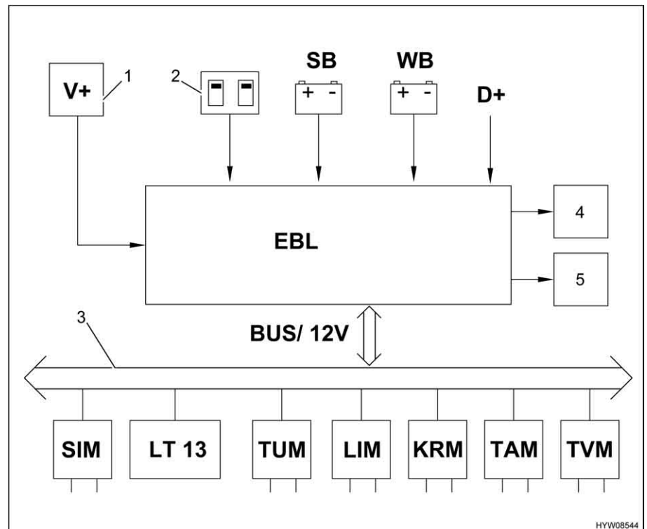
Fig. 116 Sistema a blocchi 12 V
