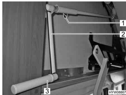
Fig. 59 Manovella per esercizio di emergenza
