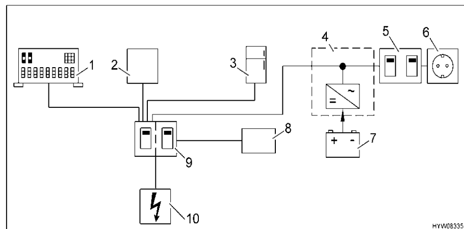
Fig. 115 Schema del cablaggio a 230 V (con invertitore)
