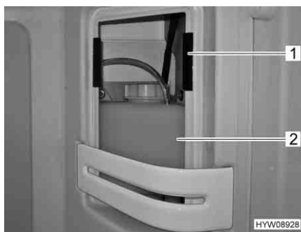
Fig. 158 Vaso d'espansione del riscaldamento ad acqua calda
