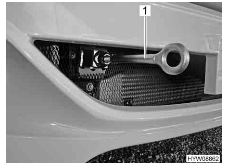
Fig. 34 Occhione di traino, installato
