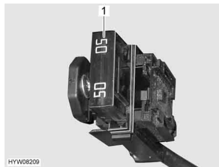
Fig. 107 Fusibili nella batteria di avviamento
