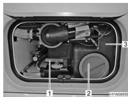
Fig. 153 Serbatoio fecale aggiuntivo
