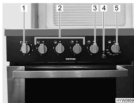
Fig. 153 Elementi di comando del blocco cucina
