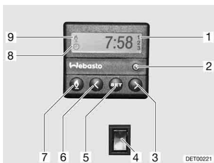
Fig. 142 Centralina di controllo per riscaldamento fisso
