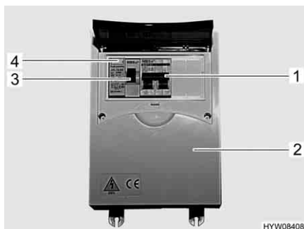
Fig. 117 Scatola dei fusibili a 230 V con interruttore di sicurezza e interruttore automatico FI
