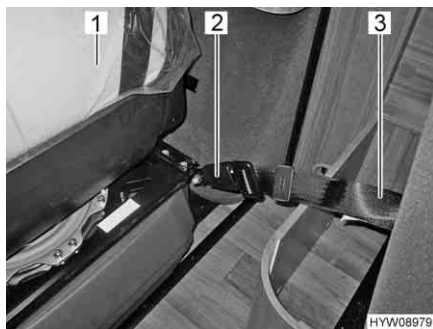
Fig. 28 Fissare il sedile installabile mediante la chiusura della cintura
