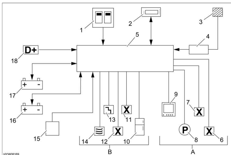
Fig. 127 Schema del cablaggio a 12 V
