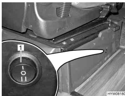
Fig. 140 Interruttore per ventola aggiuntiva
