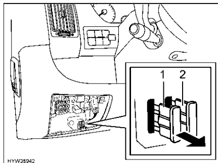
Fig. 122 Fusibili per sospensione pneumatica
