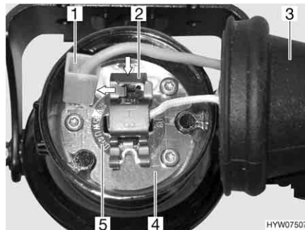
Fig. 192 Luce fendinebbia
