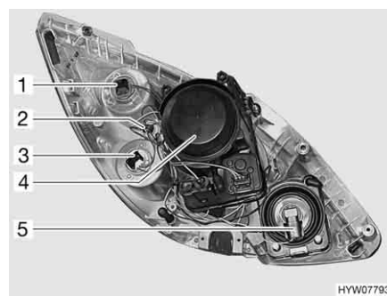
Fig. 191 Fari anteriori (lato posteriore)
