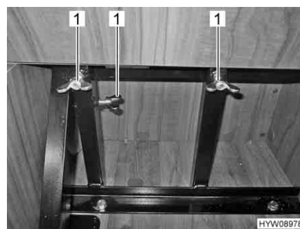
Fig. 27 Fissare il sedile installabile mediante dadi ad alette
