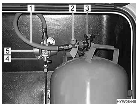
Fig. 44 Vano portabombole
