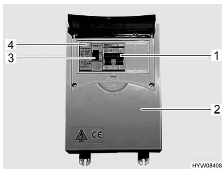
Fig. 52 Scatola dei fusibili a 230 V con interruttore di sicurezza e interruttore automatico FI
