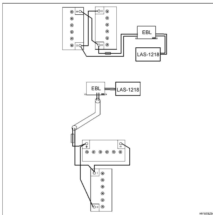
Fig. 49 Collegamento batteria ausiliare
