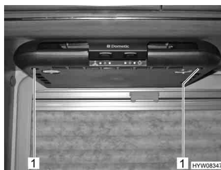
Fig. 97 Svitare la copertura inferiore
