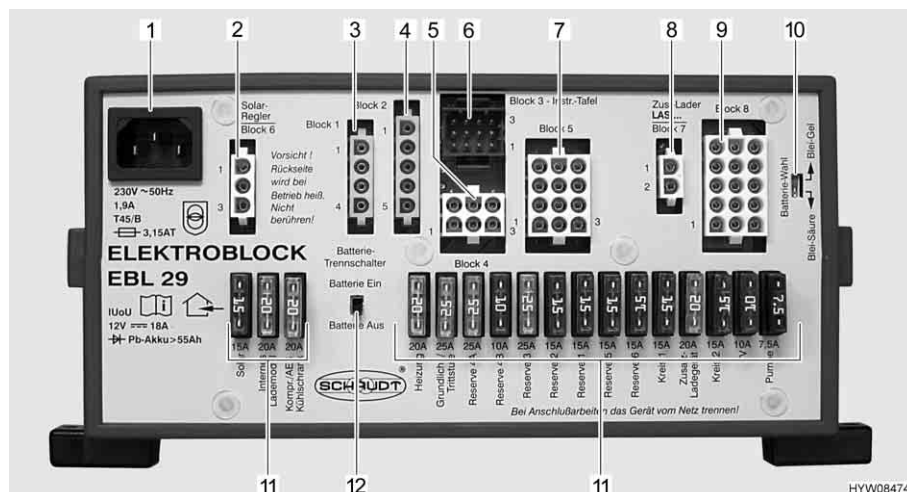
Fig. 95 Centralina elettrica (EBL 29)
