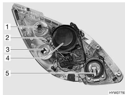
Fig. 166 Fari anteriori (lato posteriore)
