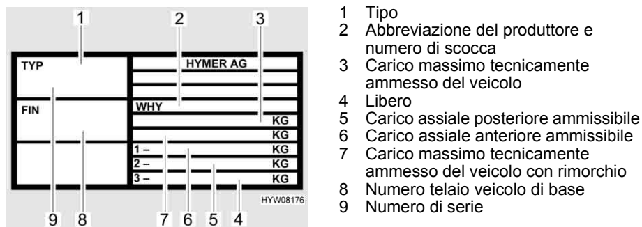
Fig. 177 Targhetta del modello
