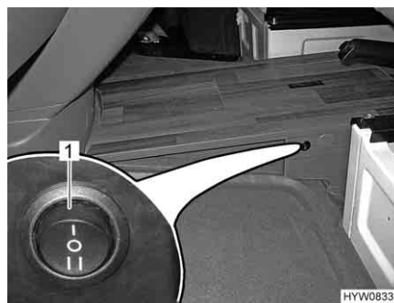
Fig. 120 Interruttore per ventola aggiuntiva (Mercedes-Benz)
