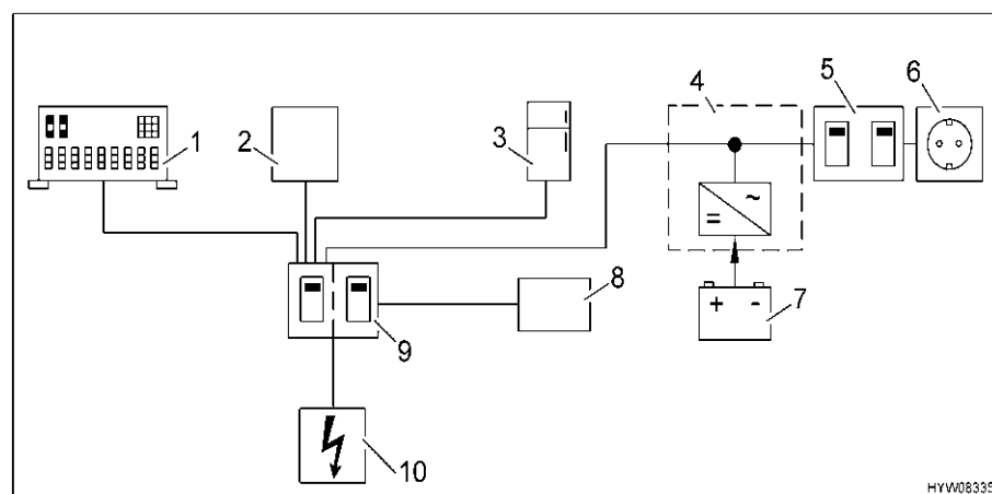
Fig. 106 Schema del cablaggio a 230 V (con invertitore)
