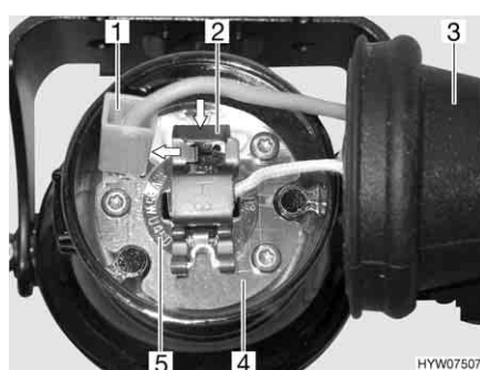
Fig. 167 Luce fendinebbia
