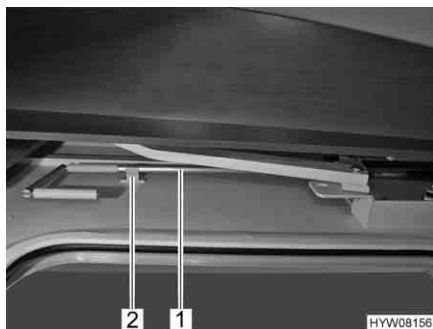
Fig. 53 Manovella per esercizio di emergenza (bloccata)
