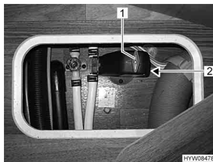
Fig. 130 Valvola di sicurezza/di scarico del boiler (alternativa)
