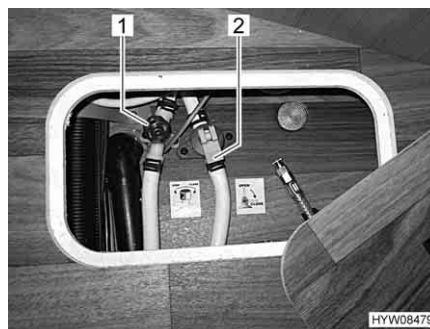
Fig. 133 Rubinetti di scarico (alternativa)
