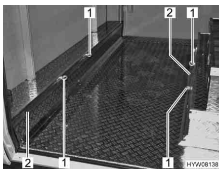
Fig. 3 Occhielli di ancoraggio garage di coda
