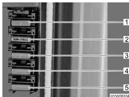
Fig. 103 Fusibili del portafusibile
