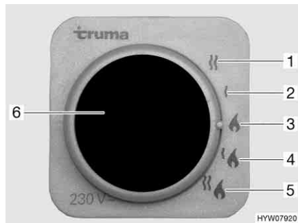
Fig. 111 Selettore di energia per riscaldamento/boiler
