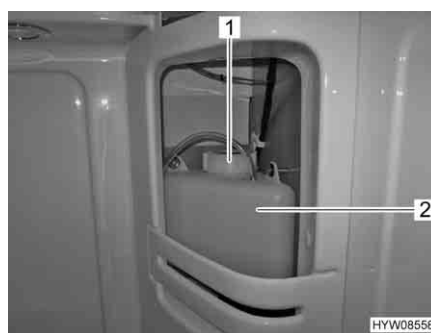
Fig. 161 Vaso d'espansione del riscaldamento ad acqua calda (vano doccia)
