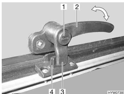
Fig. 44 Leva di serraggio in posizione "Chiuso"
