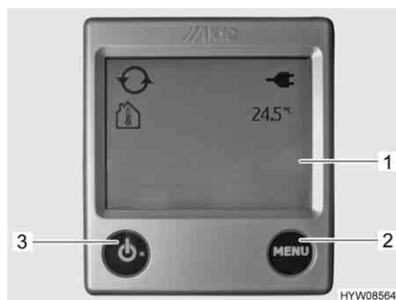
Fig. 113 Centralina di controllo, schermata iniziale per riscaldamento ad acqua calda
