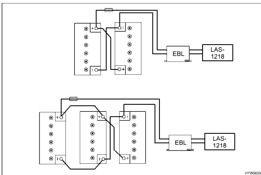
Fig. 94 Collegamento batteria ausiliare
