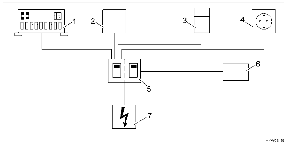
Fig. 105 Schema del cablaggio a 230 V
