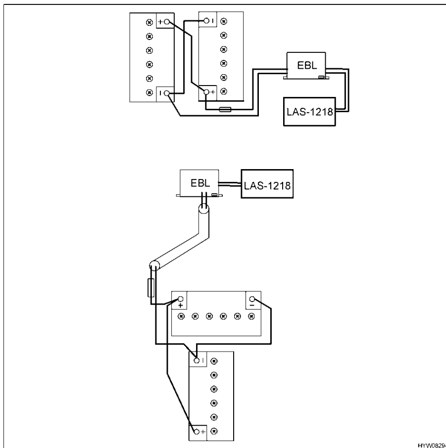
Fig. 50 Collegamento batteria ausiliare
