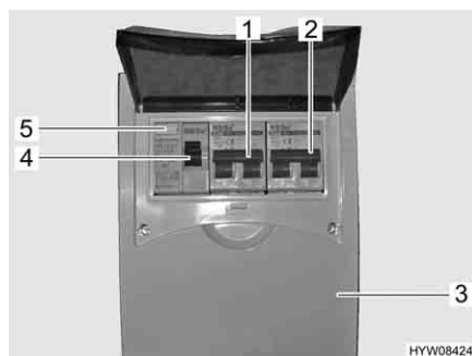
Fig. 60 Scatola dei fusibili a 230 V con interruttore di sicurezza e interruttore automatico FI
