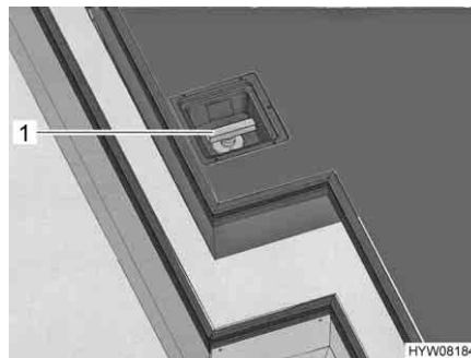
Fig. 150 Leva di comando del serbatoio delle acque grigie (alternativa)
