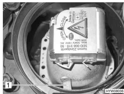
Fig. 168 Conversione fari anteriori (fari Xenon)
