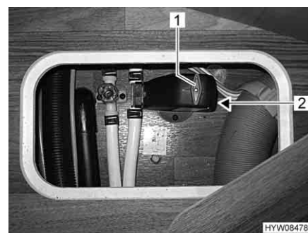
Fig. 132 Valvola di sicurezza/di scarico del boiler (alternativa)
