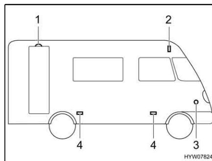
Fig. 172 Luci laterali
