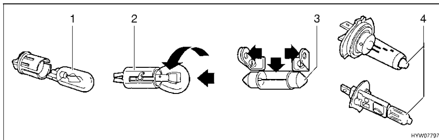
Fig. 162 Tipi di lampade ad incandescenza
