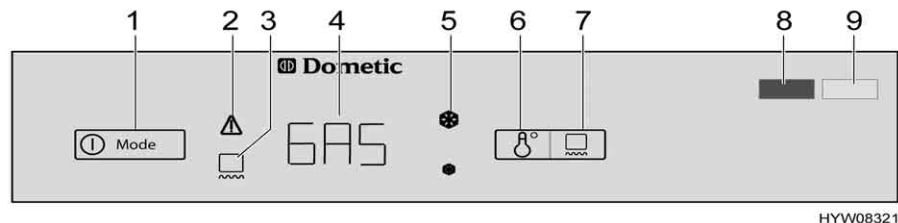
Fig. 142 Elementi di comando per il frigorifero (Dometic RMD)
