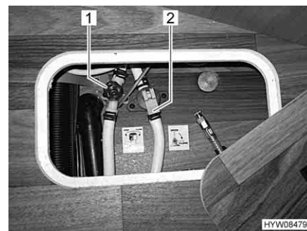
Fig. 135 Rubinetti di scarico (alternativa)
