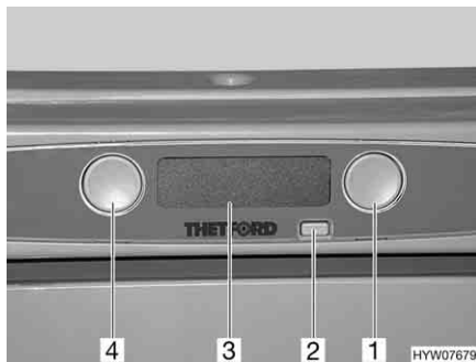
Fig. 142 Elementi di comando per il frigorifero (Thetford senza SES)
