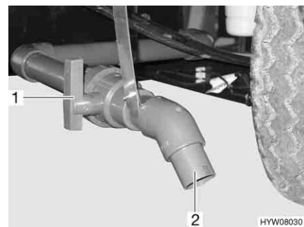
Fig. 154 Leva di comando e tubo di scarico del serbatoio delle acque grigie (alternativa)
