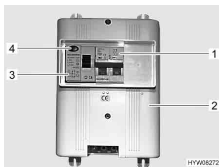
Fig. 111 Scatola dei fusibili a 230 V con interruttore di sicurezza e interruttore automatico FI
