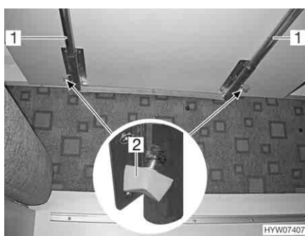
Fig. 76 Tavolo sospeso, bloccaggio della base estraibile
