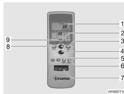
Fig. 131 Telecomando
