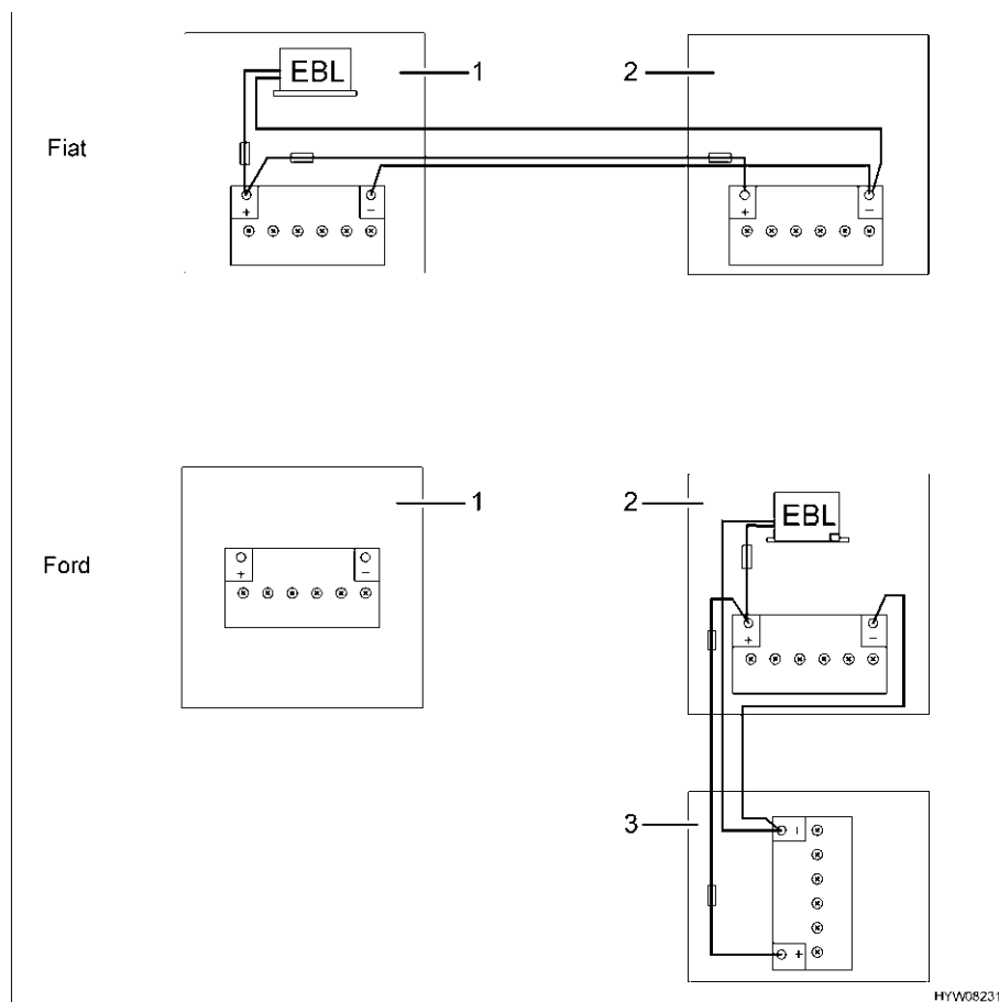
Fig. 108 Collegamento batterie ausiliarie
