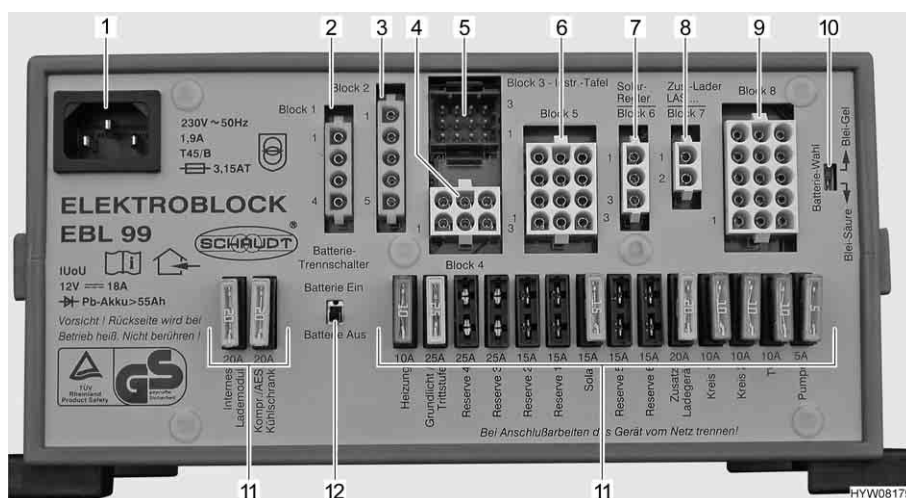
Fig. 109 Centralina elettrica (EBL 99)
