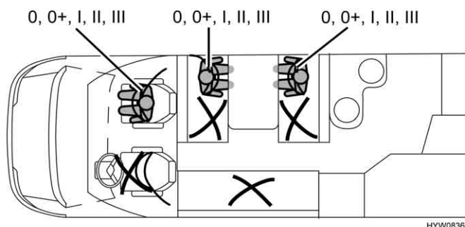
Fig. 12 Posti a sedere adatti per seggiolini per bambini (Semintegrali)
