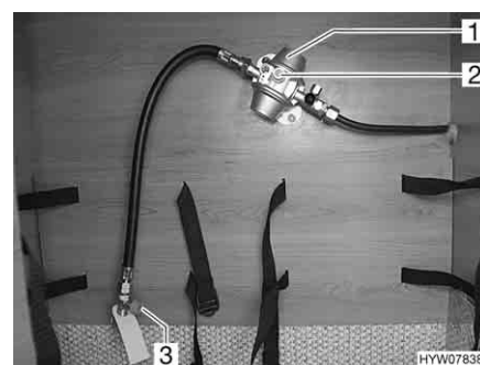
Fig. 103 Regolatore di pressione del gas
