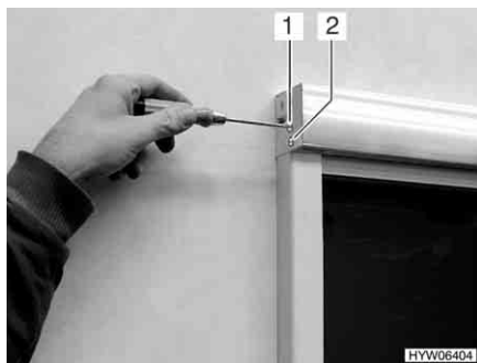
Fig. 185 Regolazione reazione elastica delle molle
