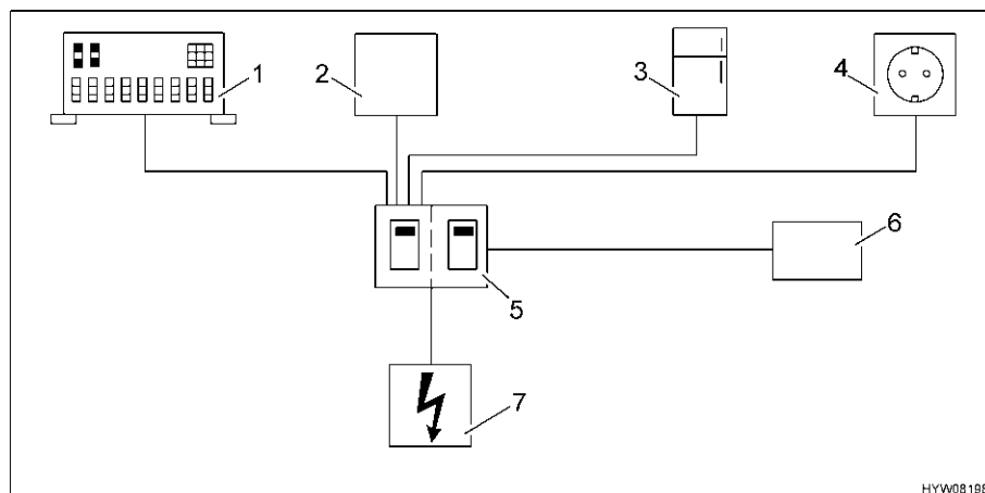
Fig. 121 Schema del cablaggio a 230 V
