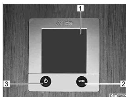
Fig. 122 Centralina di controllo per riscaldamento ad acqua calda
