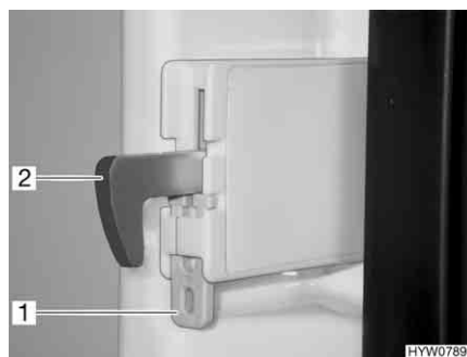
Fig. 152 Fissaggio del gancio di bloccaggio
