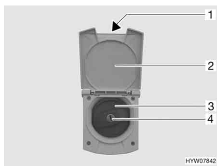
Fig. 29 Sportello e coperchio per bocchettone di riempimento dell'acqua potabile
