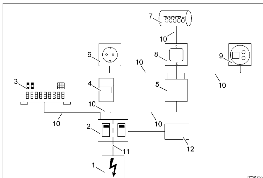
Fig. 106 Schema del cablaggio a 230 V
