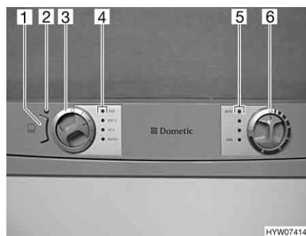
Fig. 146 Elementi di comando per il frigorifero (serie Dometic 7 con AES e RT)
