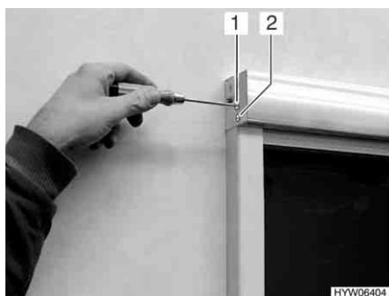
Fig. 196 Regolazione reazione elastica delle molle
