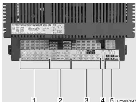
Fig. 90 Apparecchio per l'alimentazione elettrica CSV 400-1
