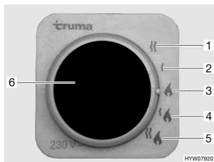
Fig. 130 Selettore di energia per riscaldamento/boiler
