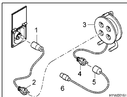
Fig. 94 Possibilità di collegamento per il collegamento a 230 V
