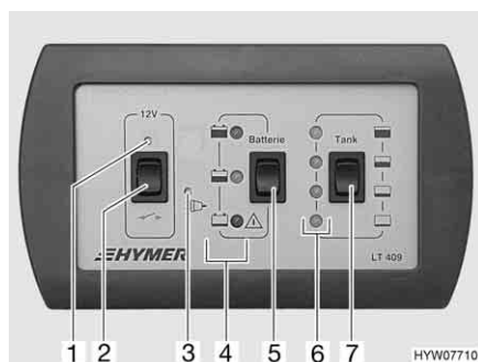
Fig. 93 Pannello di controllo LT 409
