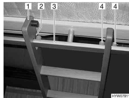
Fig. 99 Scaletta di accesso, agganciata
