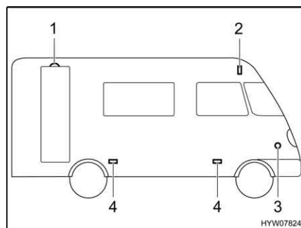
Fig. 250 Luci laterali
