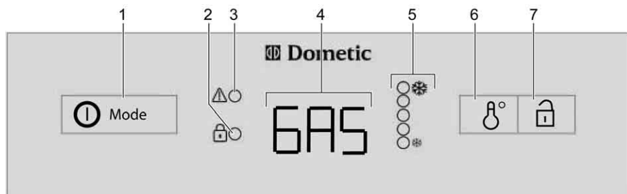
Fig. 191 Elementi di comando per il frigorifero (serie Dometic 8 con AES)
