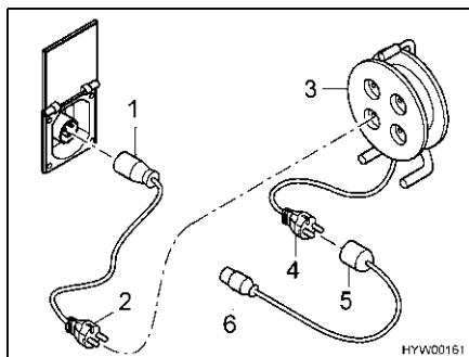
Fig. 139 Possibilità di collegamento per il collegamento a 230 V
