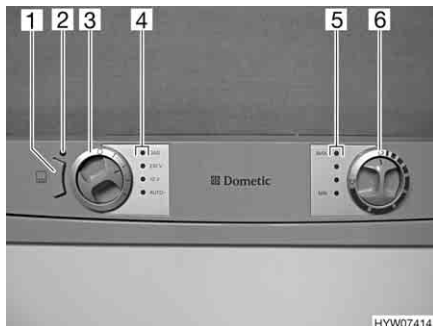
Fig. 189 Elementi di comando del frigorifero (serie Dometic 7 con AES e RT)
