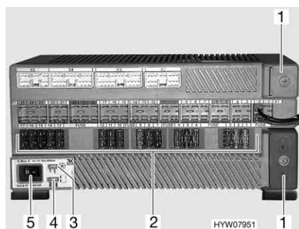
Fig. 127 Centralina elettrica (E-Box II)
