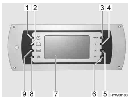
Fig. 132 Pannello di controllo (DT 202)
