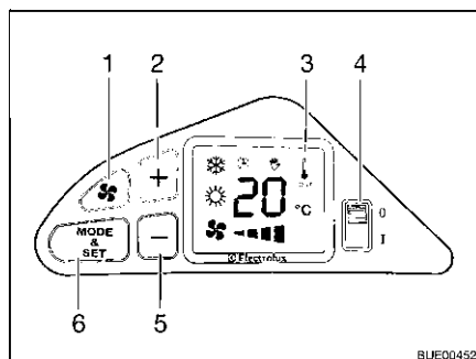
Fig. 172 Elementi di comando
