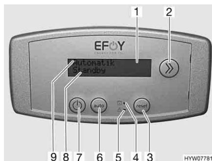
Fig. 130 Centralina di controllo per pila a combustibile
