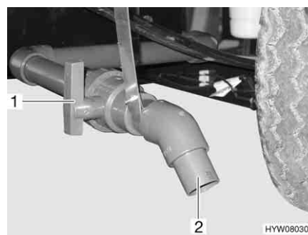
Fig. 212 Leva di comando e tubo di scarico del serbatoio delle acque grigie (alternativa)
