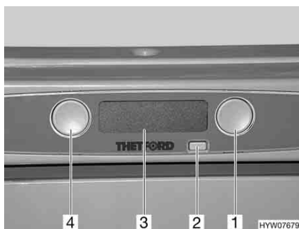
Fig. 192 Elementi di comando per il frigorifero (Thetford senza SES)
