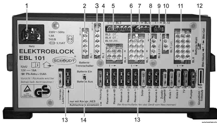
Fig. 126 Centralina elettrica (EBL 101)
