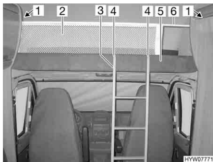
Fig. 102 Mansarda con scaletta di accesso e rete protettiva montata
