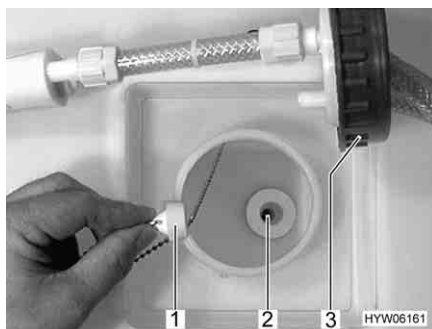
Fig. 210 Serbatoio dell'acqua
