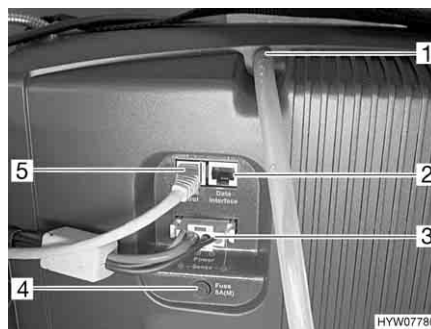
Fig. 129 Campo di collegamento pila a combustibile
