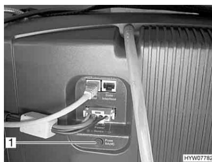
Fig. 146 Fusibile della pila a combustibile
