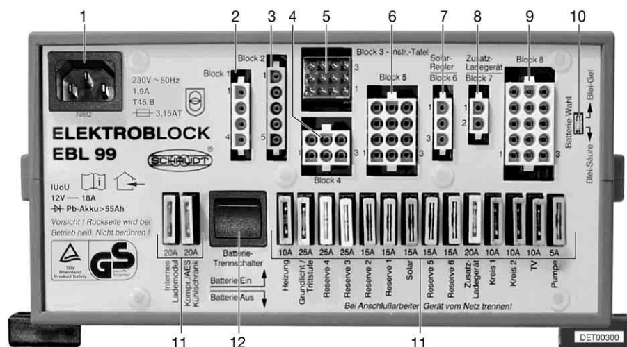
Fig. 125 Centralina elettrica (EBL 99)
