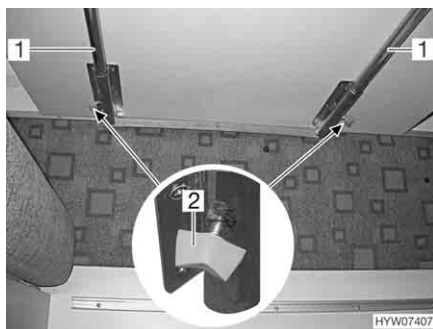
Fig. 84 Tavolo sospeso, bloccaggio della base estraibile
