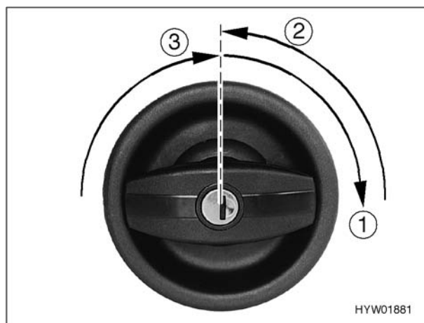
Fig. 10 Serratura della porta di ingresso, lato esterno, apertura
