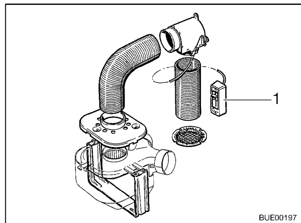
Fig. 83 Pacchetto comfort Airmix
