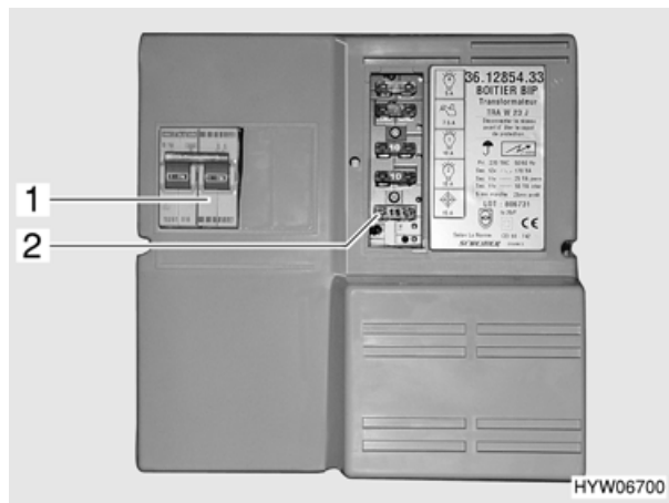
Fig. 58 Interruttore di sicurezza a 230 V con alimentatore di rete
