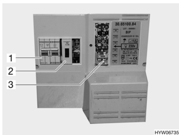
Fig. 63 Interruttore di sicurezza a 230 V (pacchetto autarchico)
