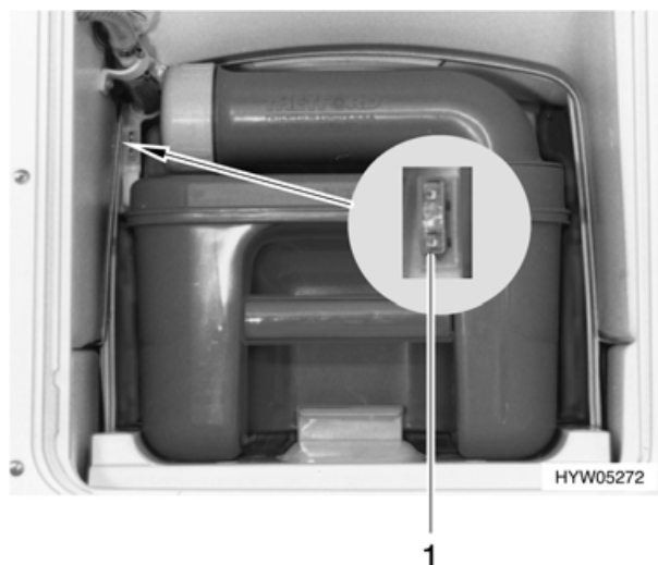
Fig. 61 Fusibile per cassetta Thetford
