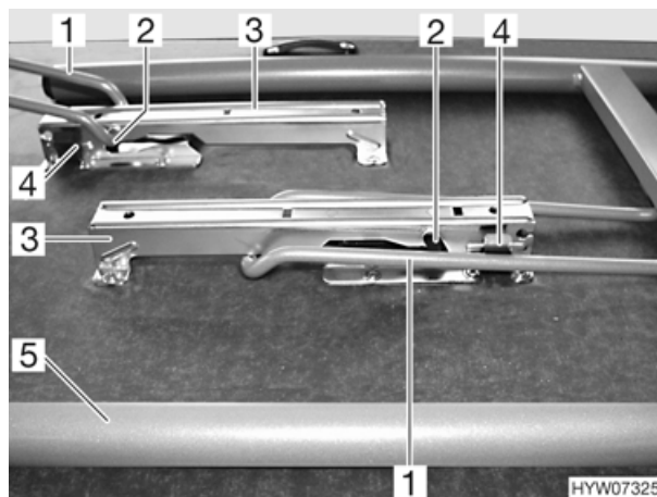
Fig. 26 Tavolo ribaltabile, meccanismo di ribaltamento
