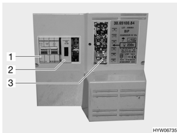
Fig. 59 Interruttore di sicurezza a 230 V con alimentatore di rete (pacchetto autarchico)
