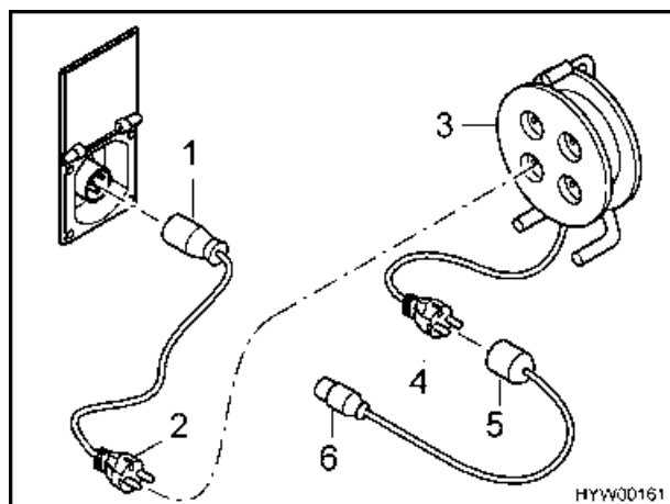
Fig. 60 Possibilità di collegamento a 230 V
