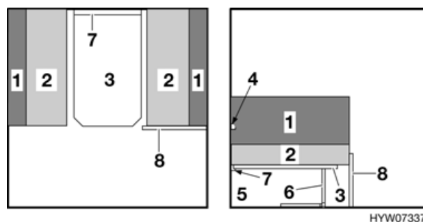
Fig. 34 Durante la trasformazione (Troll 530)
