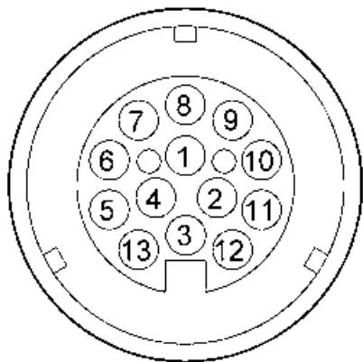
Fig. 66 Figura del contatto della spina a 13 poli
