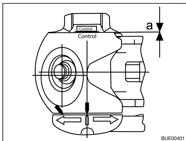
Fig. 92 Controllo usura
