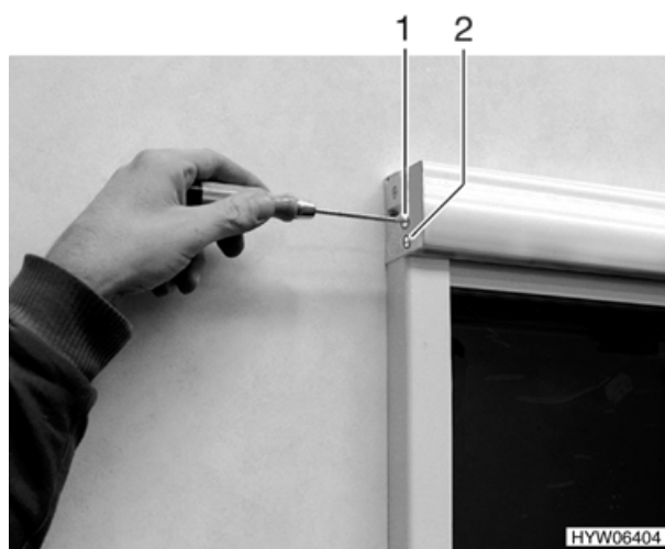
Fig. 99 Regolazione reazione elastica delle molle
