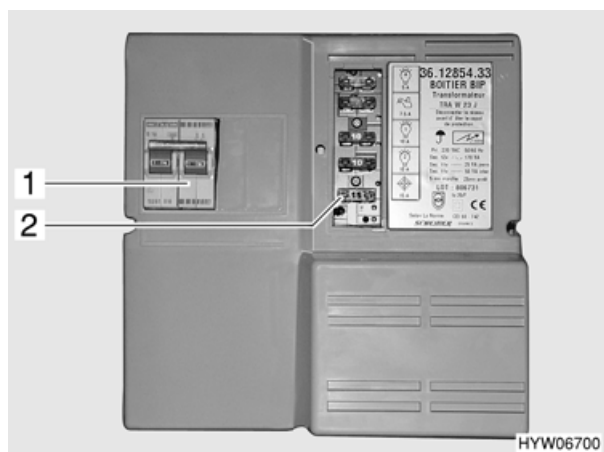
Fig. 62 Interruttore di sicurezza a 230 V
