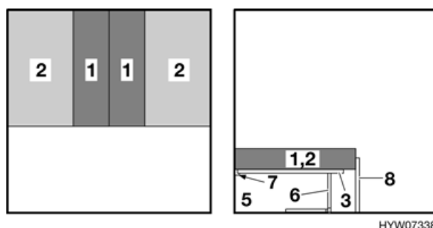
Fig. 36 Dopo la trasformazione (Troll 530)
