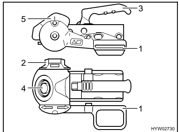
Bild 3 Anhängerkupplung Kober AK 1300 (SA)
