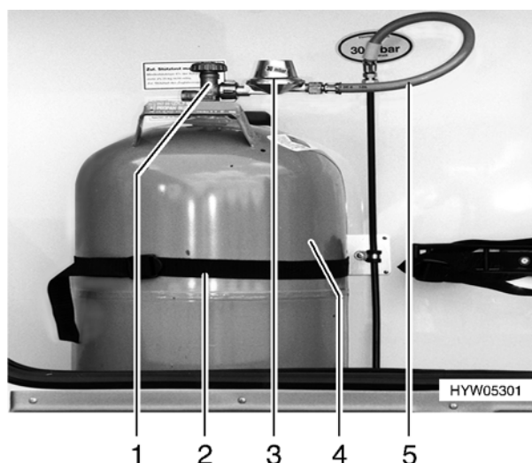
Bild 48 Gaskasten
