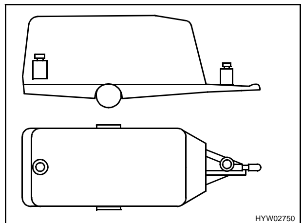
Bild 5 Falsche Gewichtsverteilung
