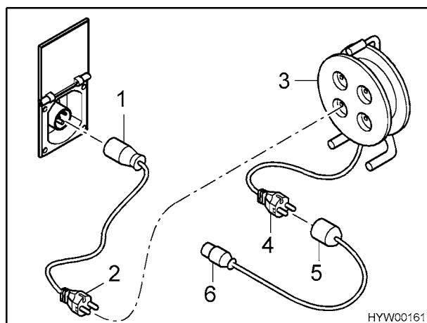
Bild 53 Außenanschluss
