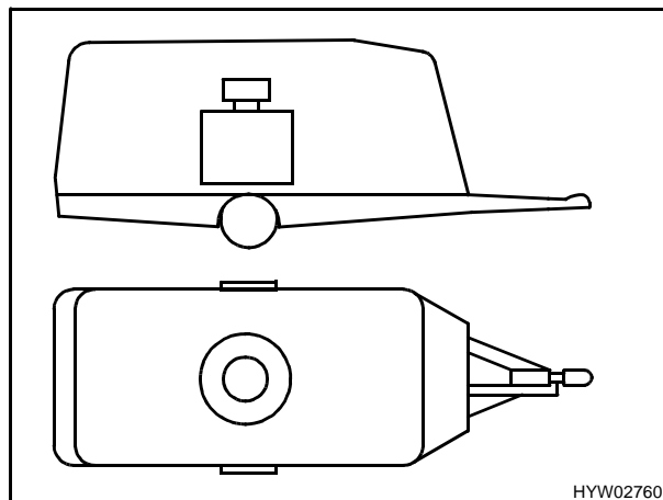
Bild 6 Richtige Gewichtsverteilung
