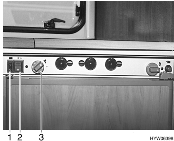
Bild 63 Bedienelemente für Kühlschrank (elektrischer Betrieb)
