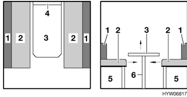
Bild 39 Vor dem Umbau
