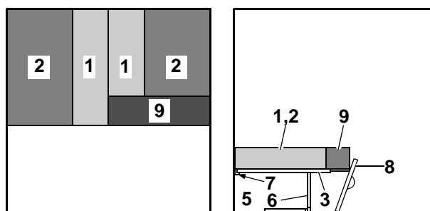
Bild 28 Nach dem Umbau (Familia, Triton Q, Triton O)
