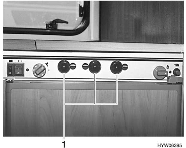
Bild 60 Bedienelemente für Gaskocher
