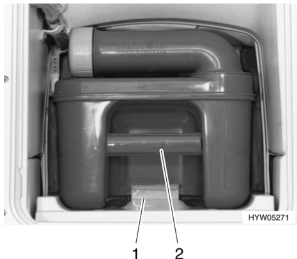
Bild 66 Thetford-Cassette entnehmen
