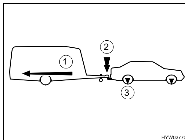
Bild 7 Anhänge-, Stütz-, Achslaster
