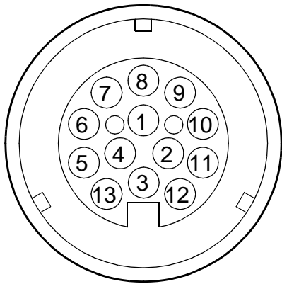
Bild 54 Kontaktbild des dreizehnpoligen Steckers
