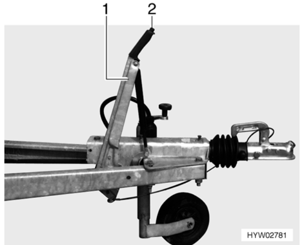
Bild 9 Feststellbremse
