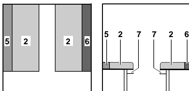
Bild 35 Nach dem Umbau
