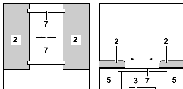
Bild 43 Während des Umbaus
