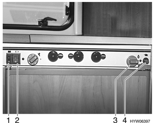
Bild 62 Bedienelemente für Kühlschrank (Gasbetrieb)
