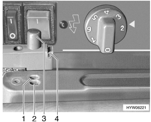
Bild 64 Arretierung der Kühlschranktür
