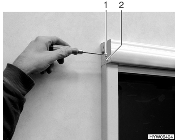
Bild 72 Federzug nachspannen
