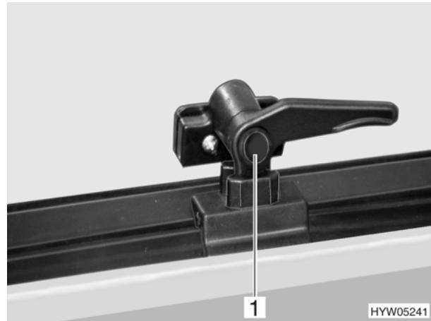
Bild 21 Ausstellfenster in Stellung Dauerbelüftung
