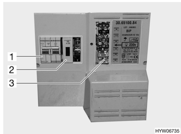
Bild 52 Netzgerät (Autark-Paket)
