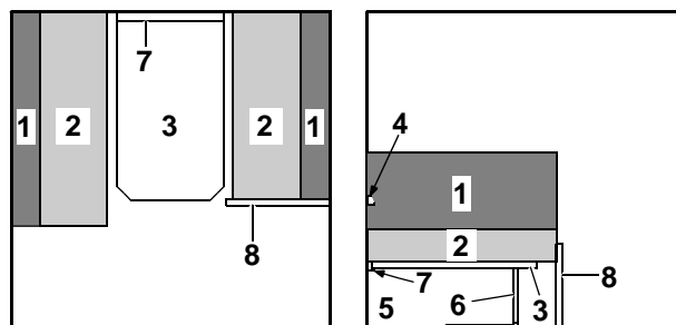
Bild 26 Während des Umbaus (Troll T)
