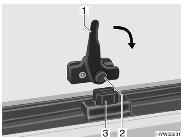
Bild 20 Ausstellfenster, Verriegelungshebel geöffnet
