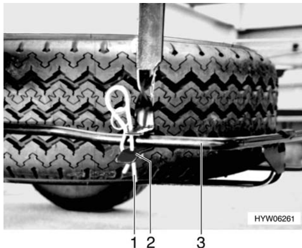
Bild 85 Ersatzrad Unterflur, seitlich
