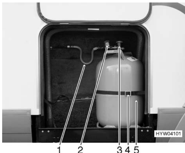
Bild 44 Gaskasten
