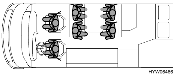
Bild 4 Sitzplatzanordnung B 544
