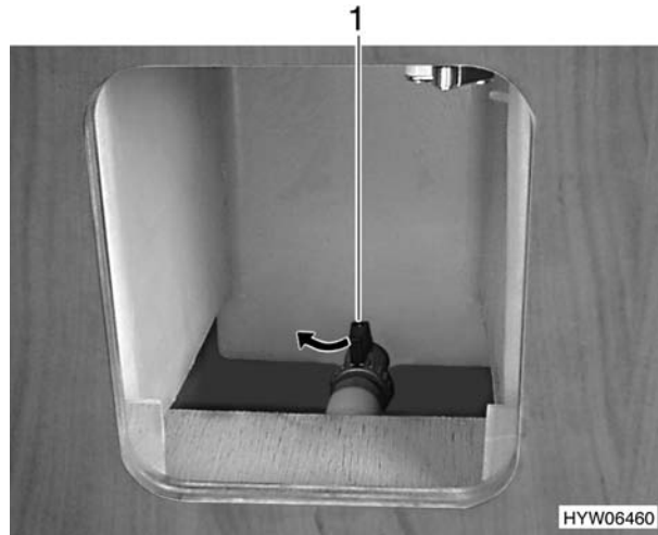
Bild 67 Frischwassertank, Wasserablaßhahn (B 584), geöffnet
