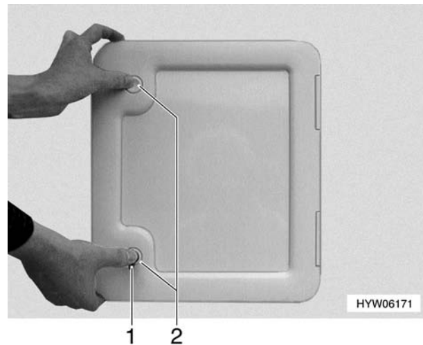
Bild 72 Öffnen der Thetford-Klappe
