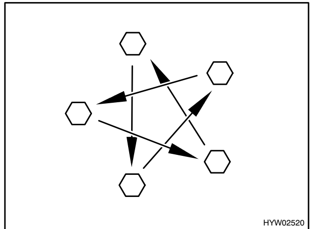
Bild 84 Radmuttern über Kreuz nachziehen
