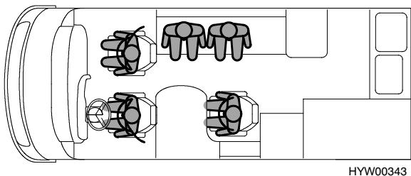
Bild 5 Sitzplatzanordnung B 584
