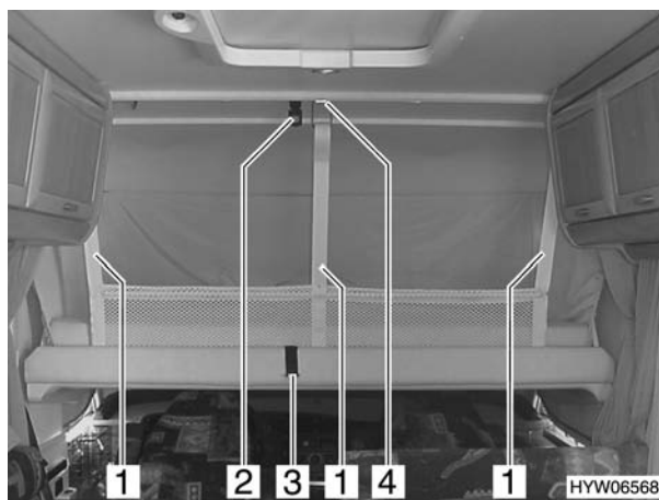
Bild 35 Hubbett mit aufgespanntem Sicherungsnetz
