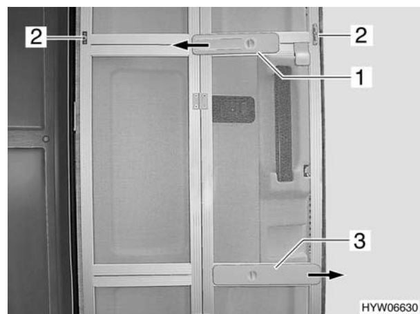
Bild 12 Mückenschutztür, ausgeklappt
