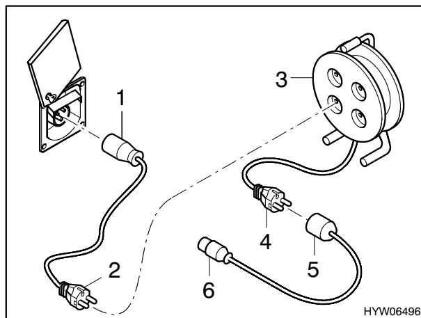
Bild 51 Anschlussmöglichkeiten 230-V-Anschluss
