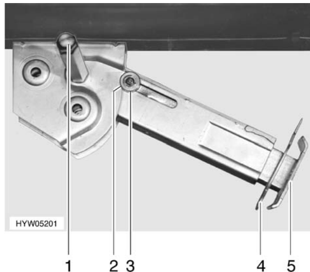
Bild 8 Hubstütze
