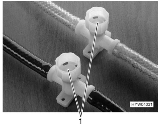
Bild 65 Ablaßventile
