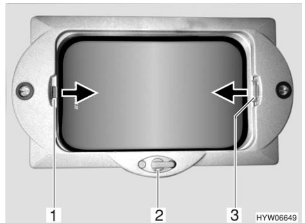
Bild 24 Kurbelhub-Dachlüfter
