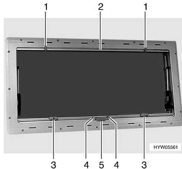
Bild 23 Ausstellfenster
