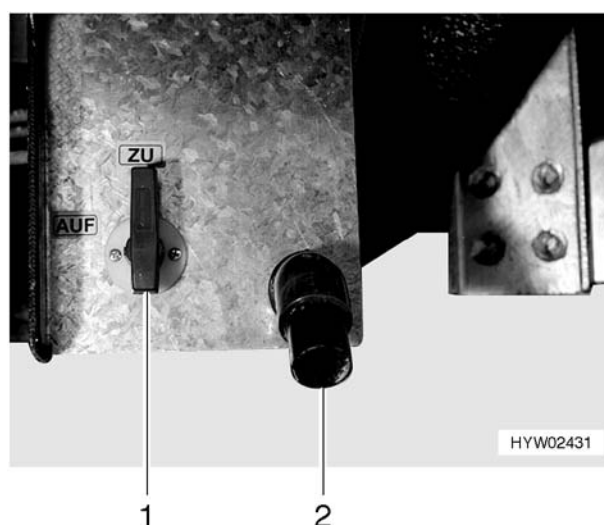
Bild 68 Bedienhebel und Ablaufrohr des Abwassertanks
