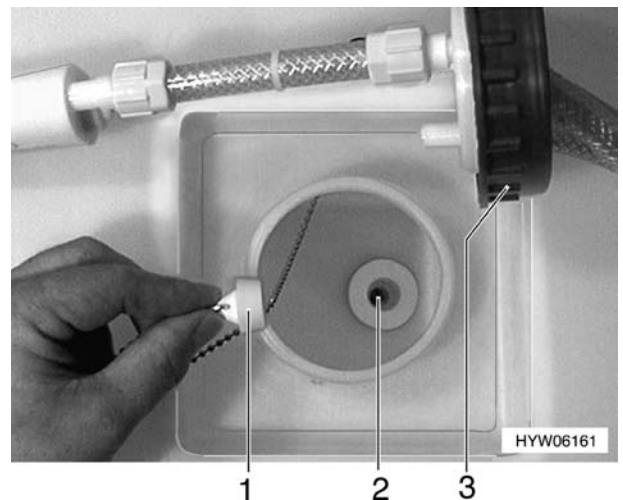
Bild 66 Frischwassertank, Verschlußstopfen (B 544)
