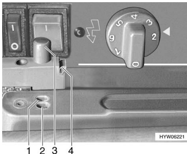
Bild 84 Verriegelung der Kühlschranktür
