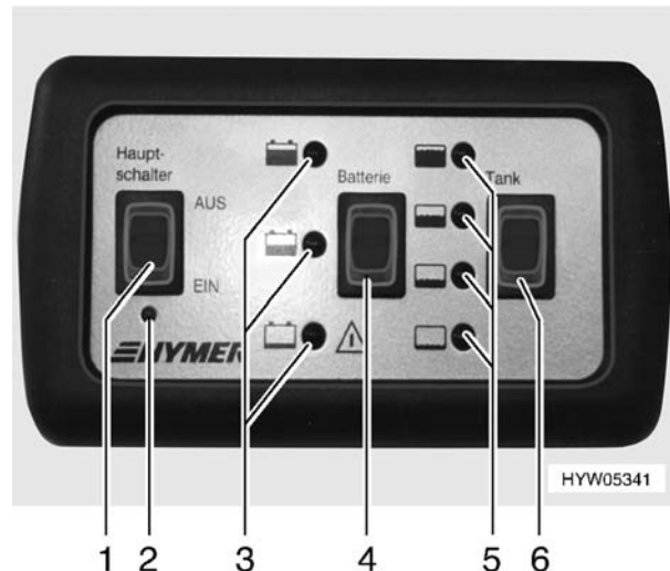
Bild 62 Panel (Moving/Autark-Paket)
