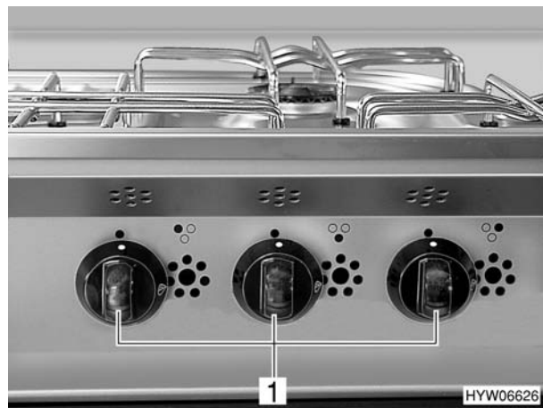
Bild 78 Bedienelemente für Gaskocher (Swing/Nova)
