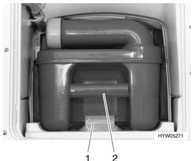
Bild 93 Thetford-Cassette entnehmen
