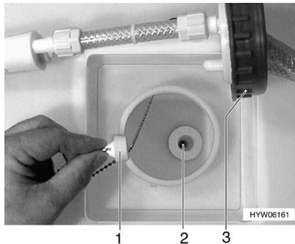
Bild 87 Frischwassertank, Verschlußstopfen
