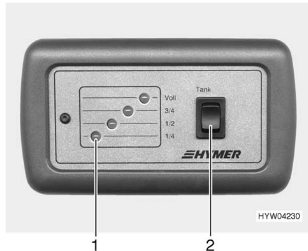
Bild 61 Panel (Swing/Nova)
