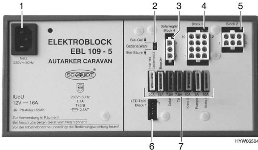
Bild 63 Elektroblock
