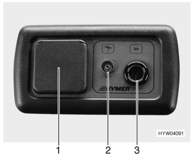
Bild 65 Steckdose
