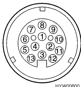
Bild 66 Steckseite der Steckdose (dreizehnpoliges System Jäger)
