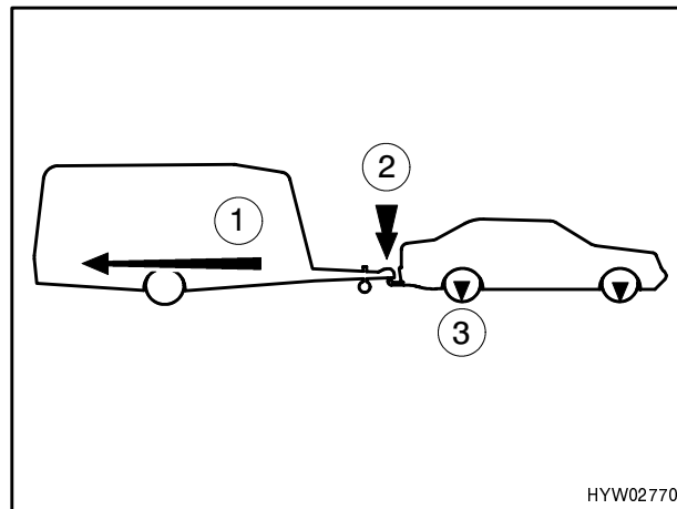
Bild 7 Anhängelast, Stütz-, Achslast
