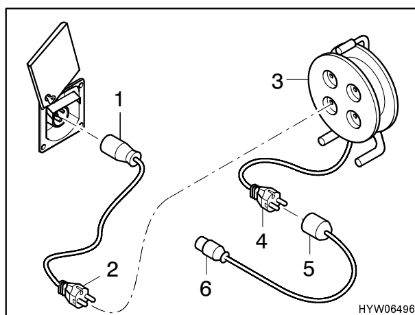
Bild 60 Außenanschluß
