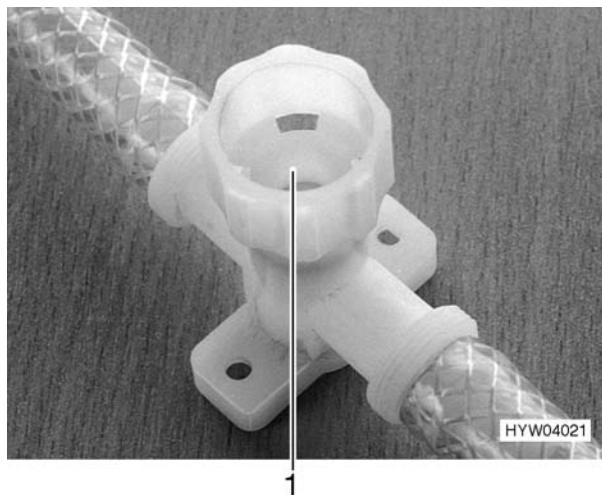
Bild 75 Ablassventil (Swing/Nova)
