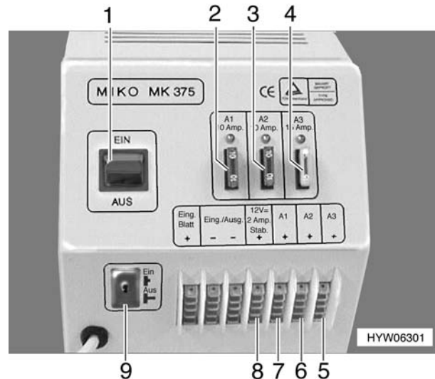
Bild 59 Netzgerät (Swing/Nova)
