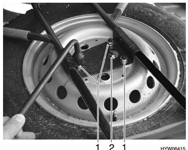
Fig. 134 Viti di fissaggio ruota di scorta
