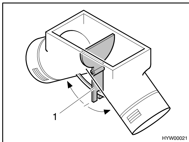
Fig. 86 Ventola di ricircolo aria Trumavent in posizione centrale
