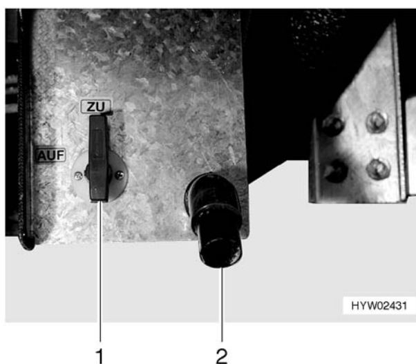
Fig. 108 Leva aperto/chiuso e tubo di scarico del serbatoio acque scure, pos. di chiuso
