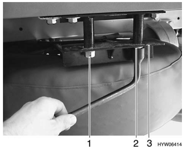
Fig. 133 Attrezzo sostegno ruota di scorta
