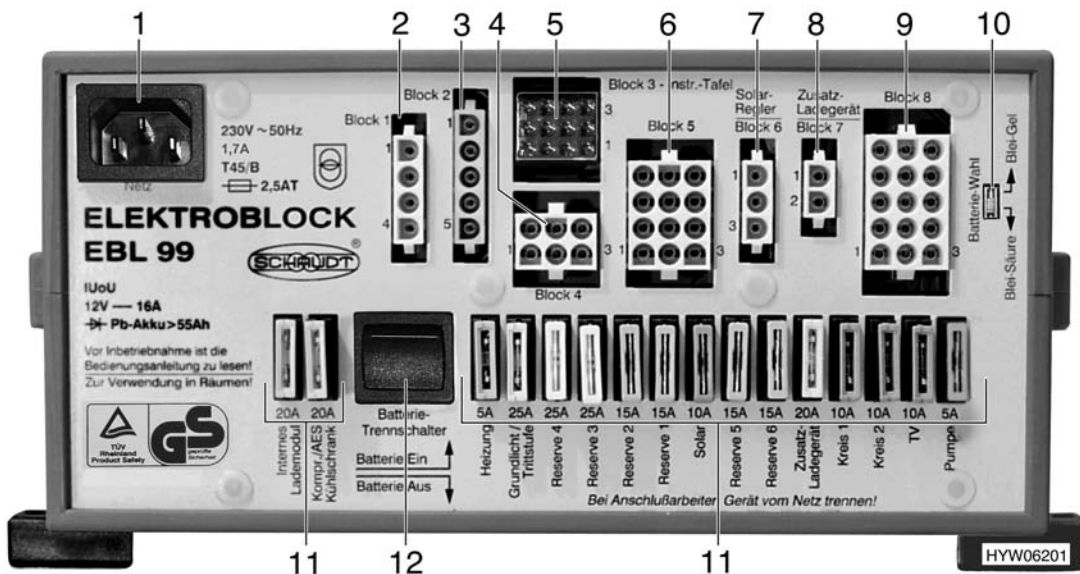
Fig. 79 Centralina elettrica EBL 99
