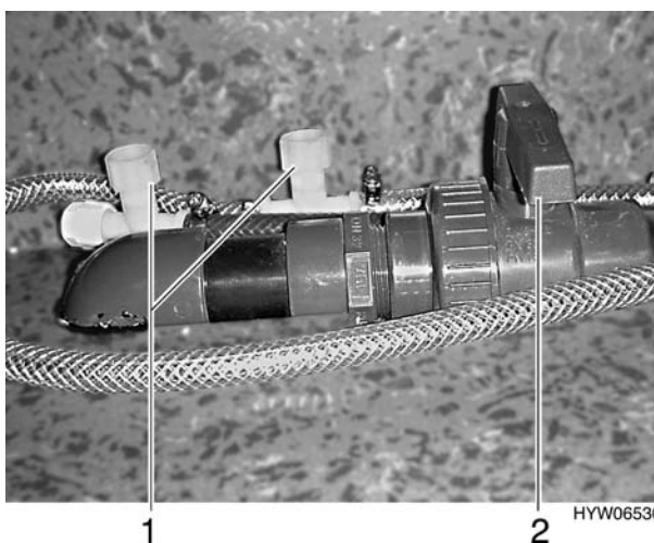
Fig. 109 Leva aperto/chiuso per serbatoio acqua scure nel garage di coda, pos. di chiuso
