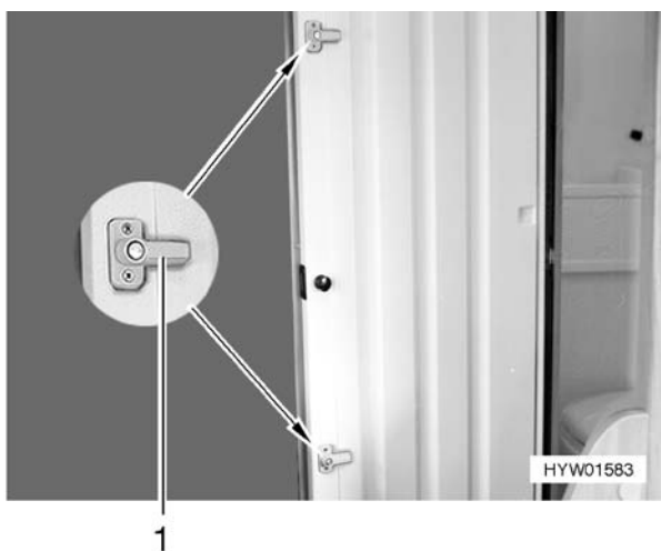
Fig. 117 Bagno Vario, porta del bagno, bloccaggio porta, parte interna
