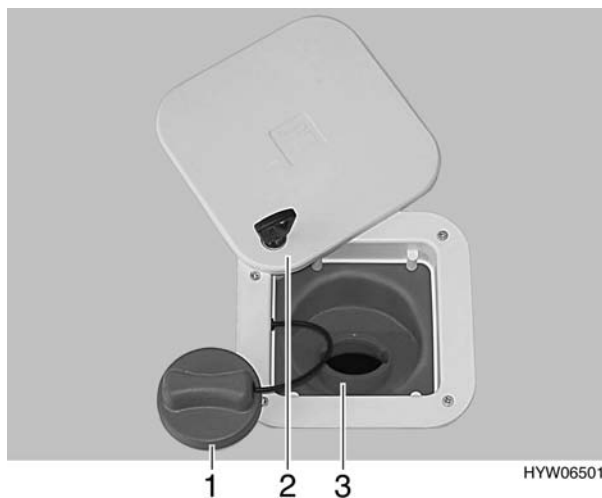
Fig. 8 Bocchettone di riempimento carburante, aperto
