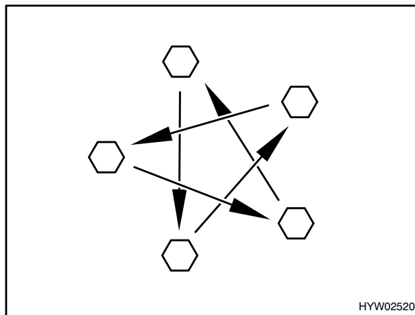
Fig. 127 Serraggio a croce dei bulloni delle ruote
