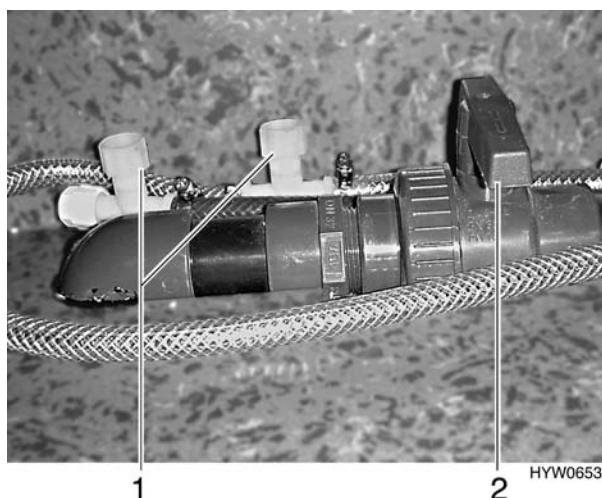
Fig. 105 Valvole di scarico per modelli con intercapedine pavimento
