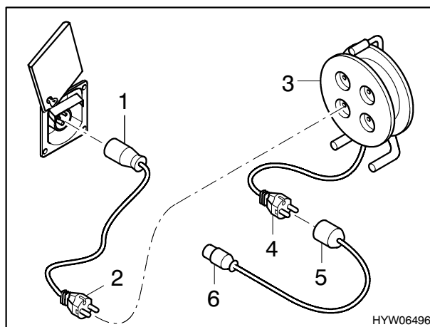
Fig. 77 Allacciamento esterno
