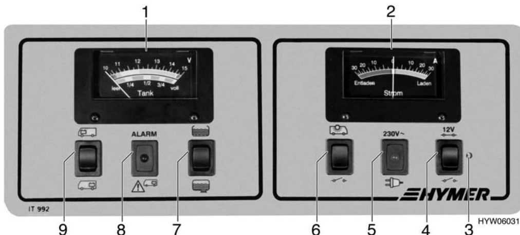
Fig. 78 Pannello
